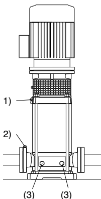
Fig. 3 (1) Remplissage et évent (2) Event aspiration (3) Vidange
