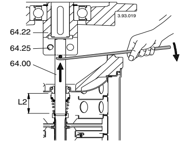
Abb. 6b Angehobener Läufer, Blockierposition Welle in Kupplung.
