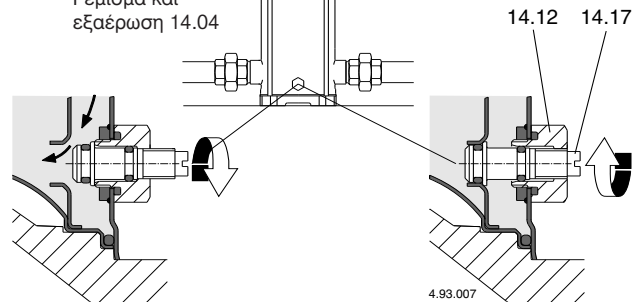
Σχ. 3a Γέμισμα: εσωτερική διόδος ανοίγματος
