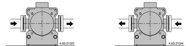
Variante 1: Saugleitung links, Durchleitung rechts
