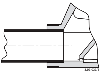
Рис. 1 Соединение приклеиванием.
