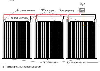
Рис. Схема подключения термоленты CALEO PLATINUM
