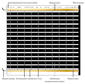
Рис. Общий вид термоленты CALEO, расположенной основными ее элементами, контактных зажимов и мест подключения к изоляции
