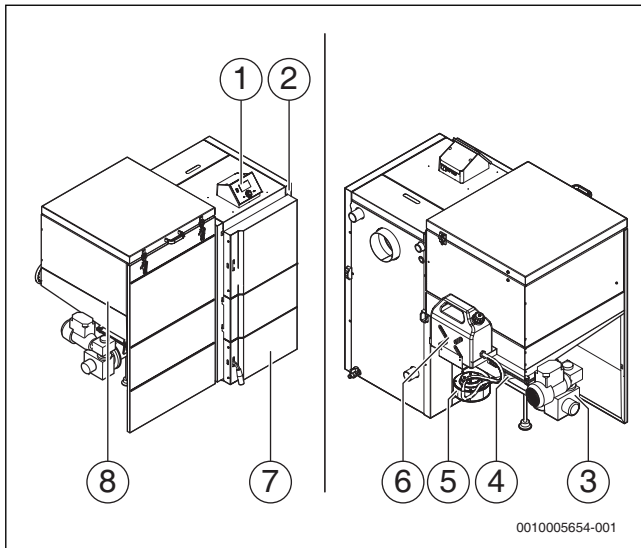
Рис. 10 Обзор котла
