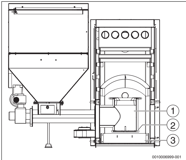
Рис. 16 Детали для очистки
