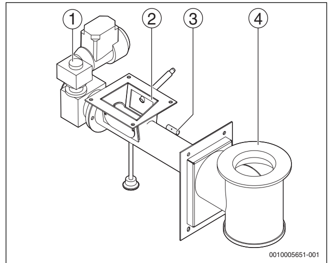
Рис. 2 Отдельные части узла горелки
