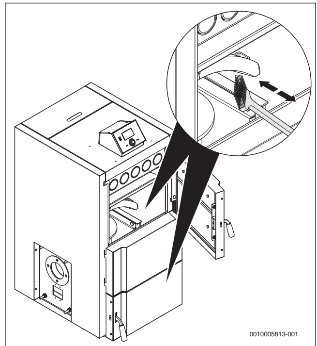
Рис. 11 Очистка топочной камеры
