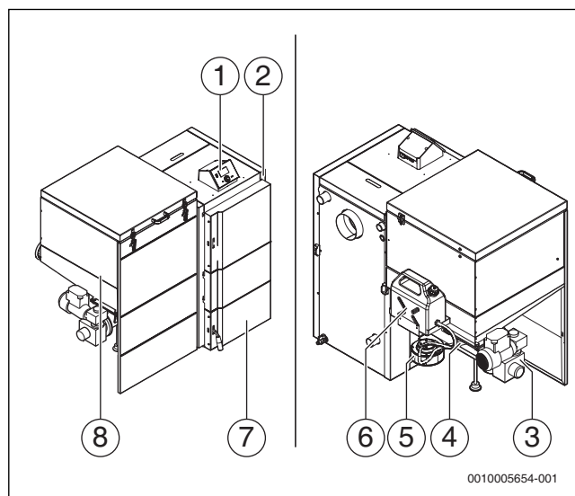
Рис. 1 Обзор котла
