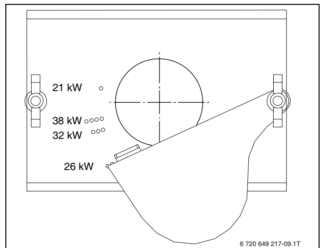
Рис 6 Регулировка заслонки вторичного воздуха по мощности котла
