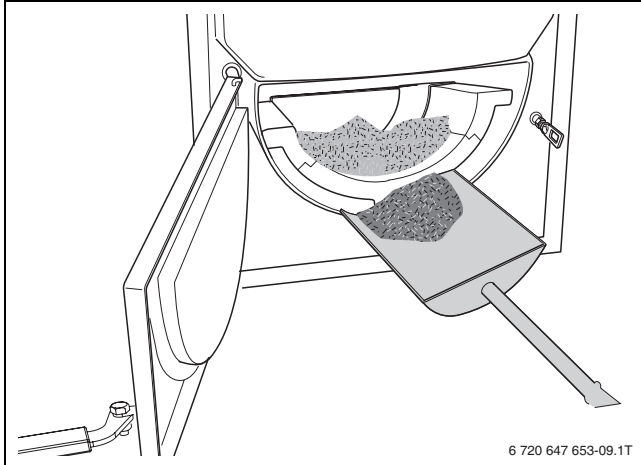
Рис 17 Удаление золы
