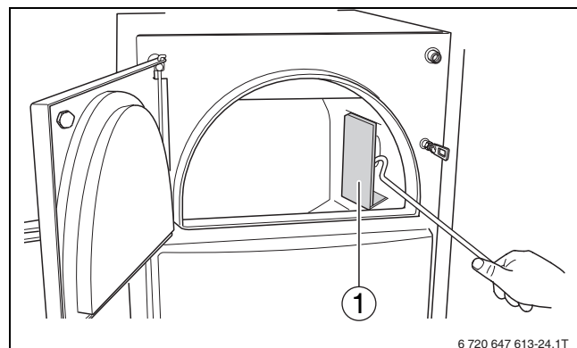
Рис 15 Проверка отверстий защитных листов
