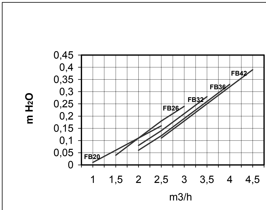
Рис. Гидравлические потери котловых корпусов (м) в зависимости от тока воды (м 3 /ч)
