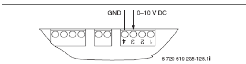
Рисунок 117 Регулирование мощности
