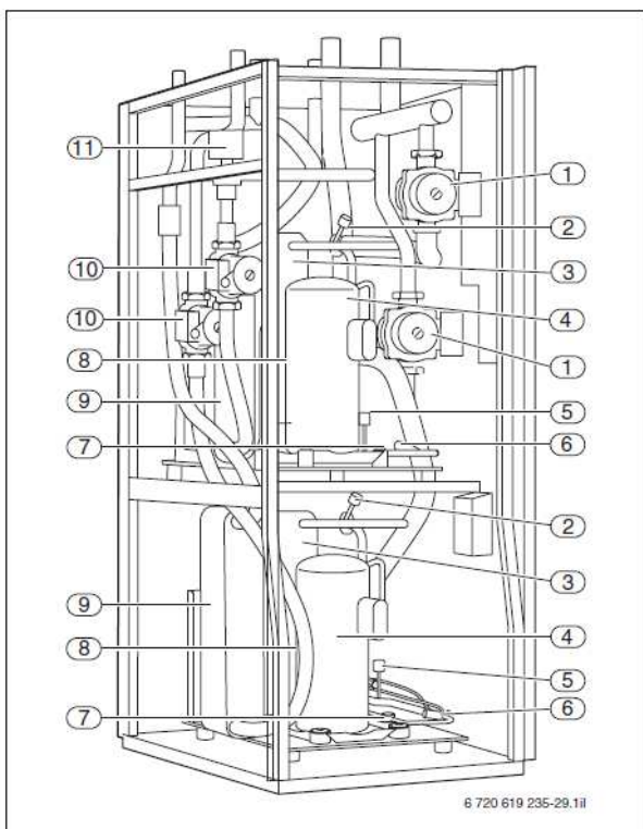
Рисунок 19 Конструкция теплового насоса Logatherm WPS 22–33
