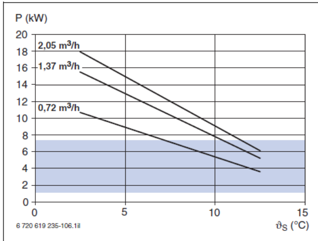
Рисунок 104 Диаграмма мощности станции пассивного охлаждения PKSt (Рабочий диапазон для WPS 6–11 К и WPS 6–17 выделен синим)
