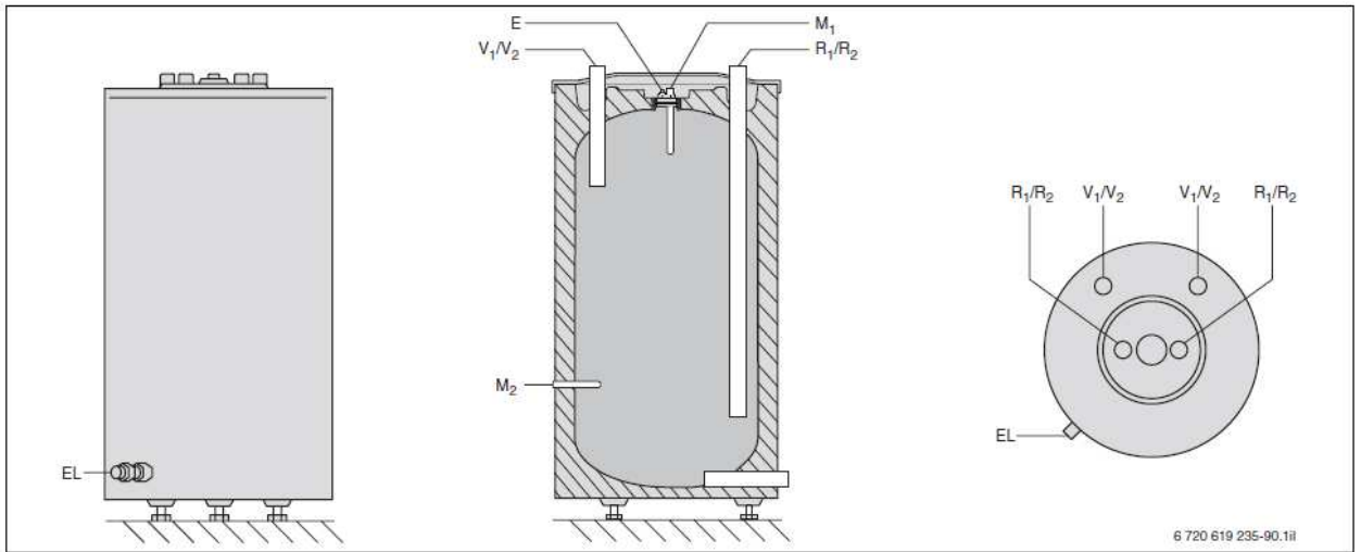
Рисунок 87 Подключение буфера P120 W
