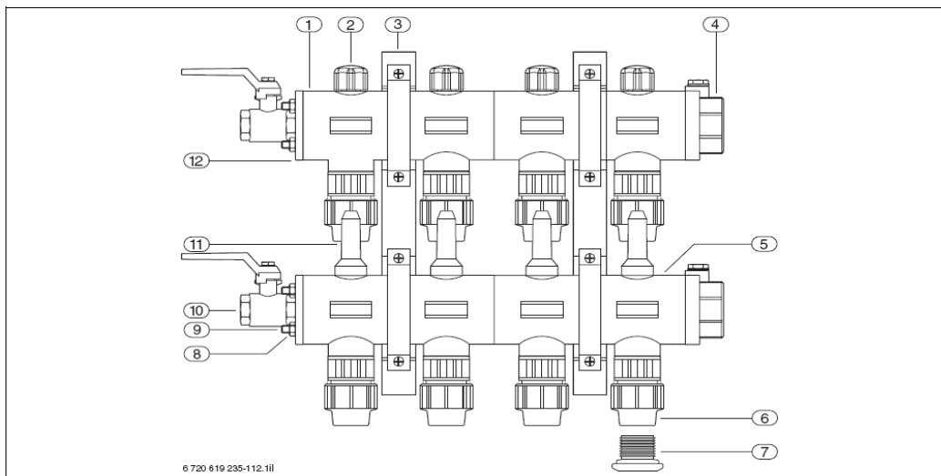
Рисунок 109 Устройство гребенки рассольного контура на примере для четырех контуров
