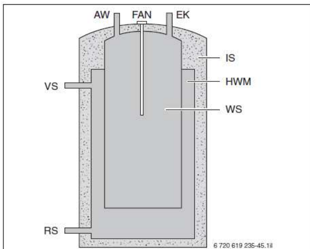
Рисунок 36 Конструкция бака-водонагревателя из высококачественной стали
