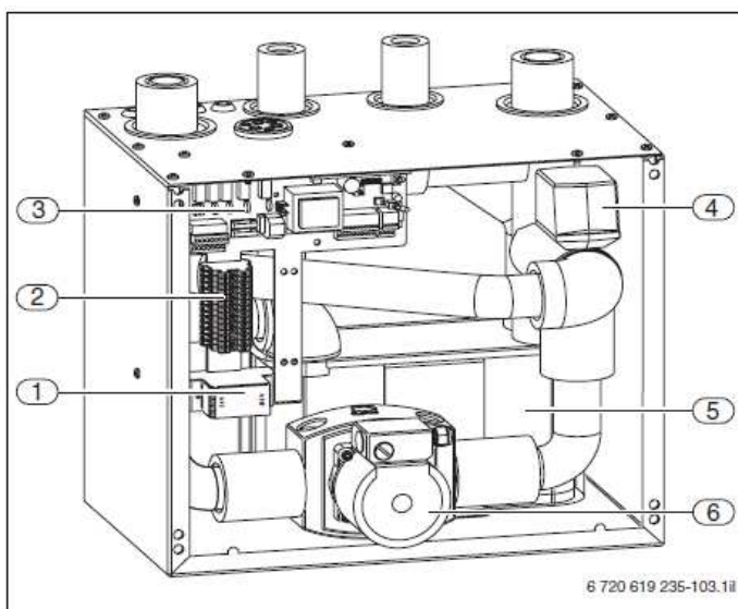
Рисунок 101 Конструкция станции пассивного охлаждения PKSt
