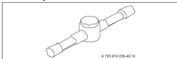
Рисунок 30 Смотровое стекло
