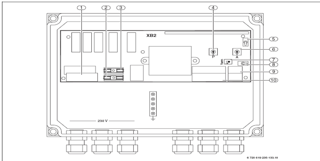
Рисунок 128 Устройство
