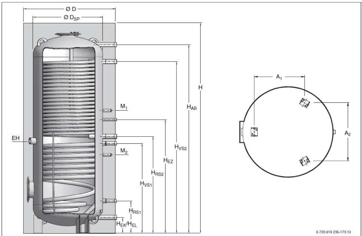
Рисунок 84 Размеры бивалентных баков SMH400 E и SMH500 E
