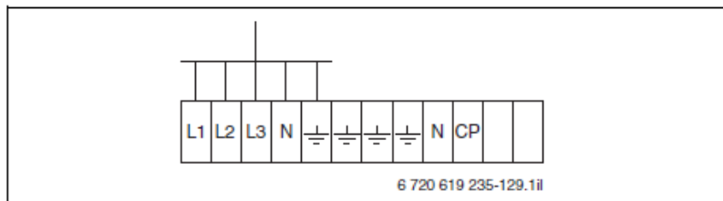
Рисунок 115 Подсоединение питающего кабеля
