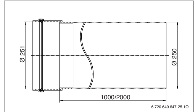
Рис. 40 Размеры в мм
