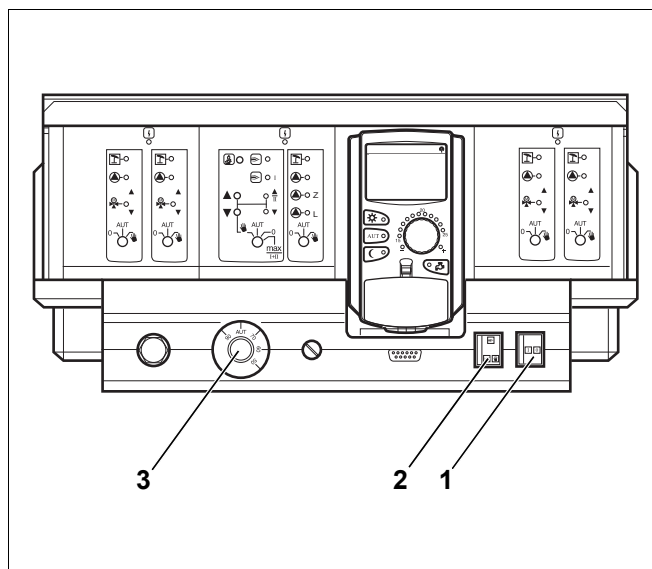
Рис. 2 Система управления Logamatic 4211
