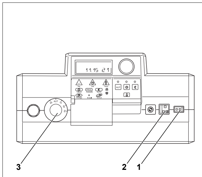
Рис. 1 Система управления Logamatic 2107
