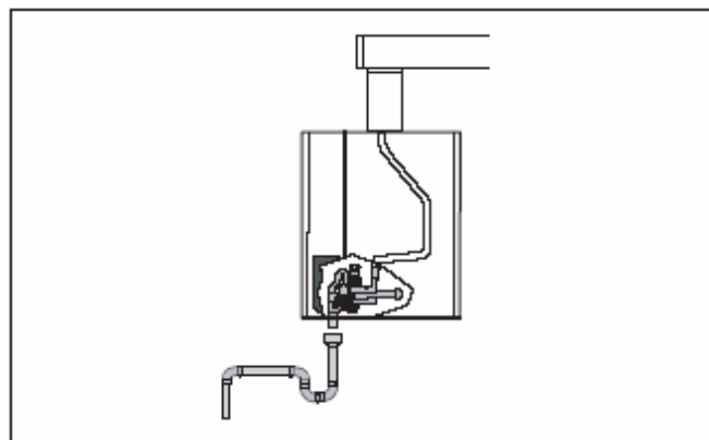
Рис. 8 Отвод конденсата из систем дымоходов, выполненных из пластмассы или нержавеющей стали
