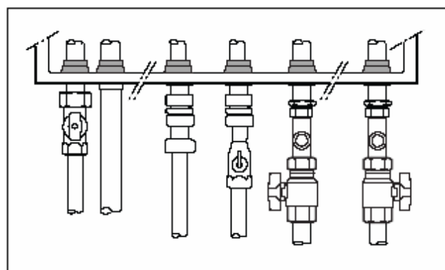
Рис. 43 Осмотр общих коррозионных проявлений
