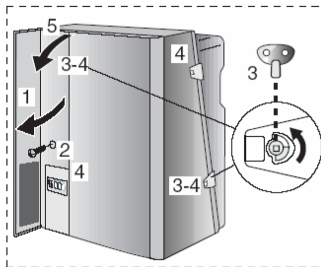
Рис. 2 Снятие обшивки
