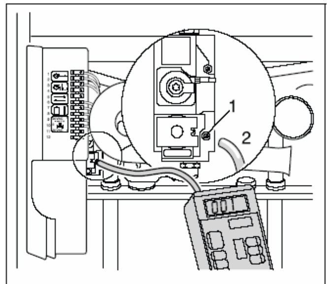
Рис. 25 Измерение давления подачи газа (арматура Honeywell)
