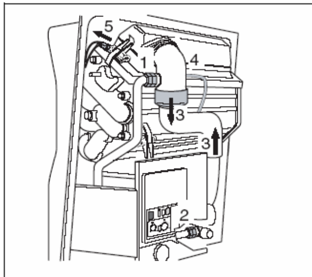
Рис. 33 Разборка присоединений
