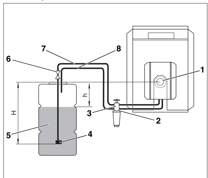
Рис. 44 Топливный бак установлен ниже топливного насоса
