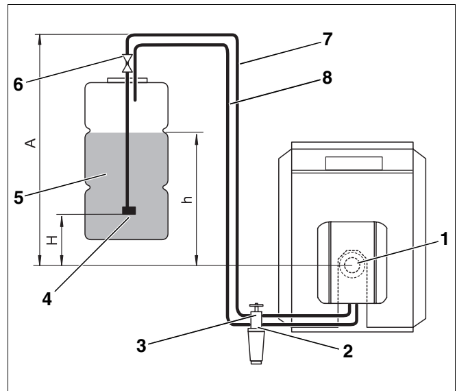
Рис. 43 Топливный бак установлен выше топливного насоса
