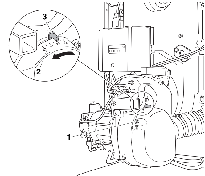
Рис. 24 Регулировка подвода всасываемого воздуха
