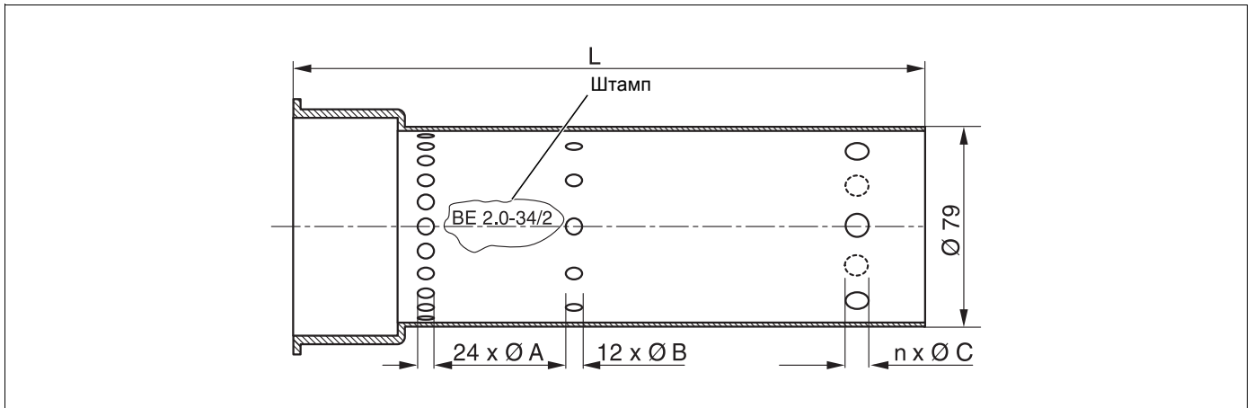
Рис. 5 Трубы горелок для чугунных и стальных котлов
