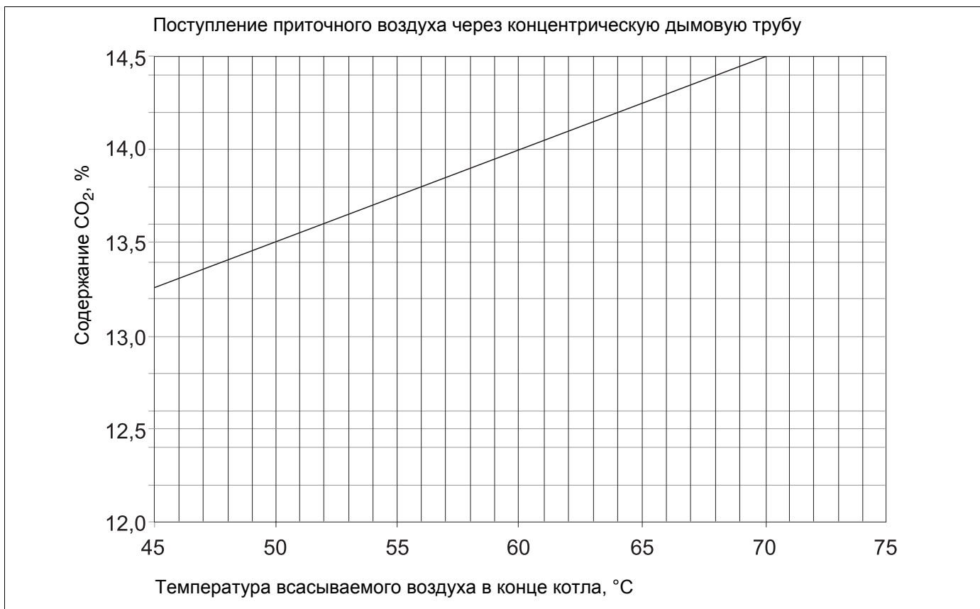
Рис. 7 Настройка CO 2 в зависимости от температуры всасываемого воздуха при поступлении его по концентрической трубе для подачи воздуха на горение и отвода дымовых газов (действительно как при наличии кожуха горелки, так и без него)
