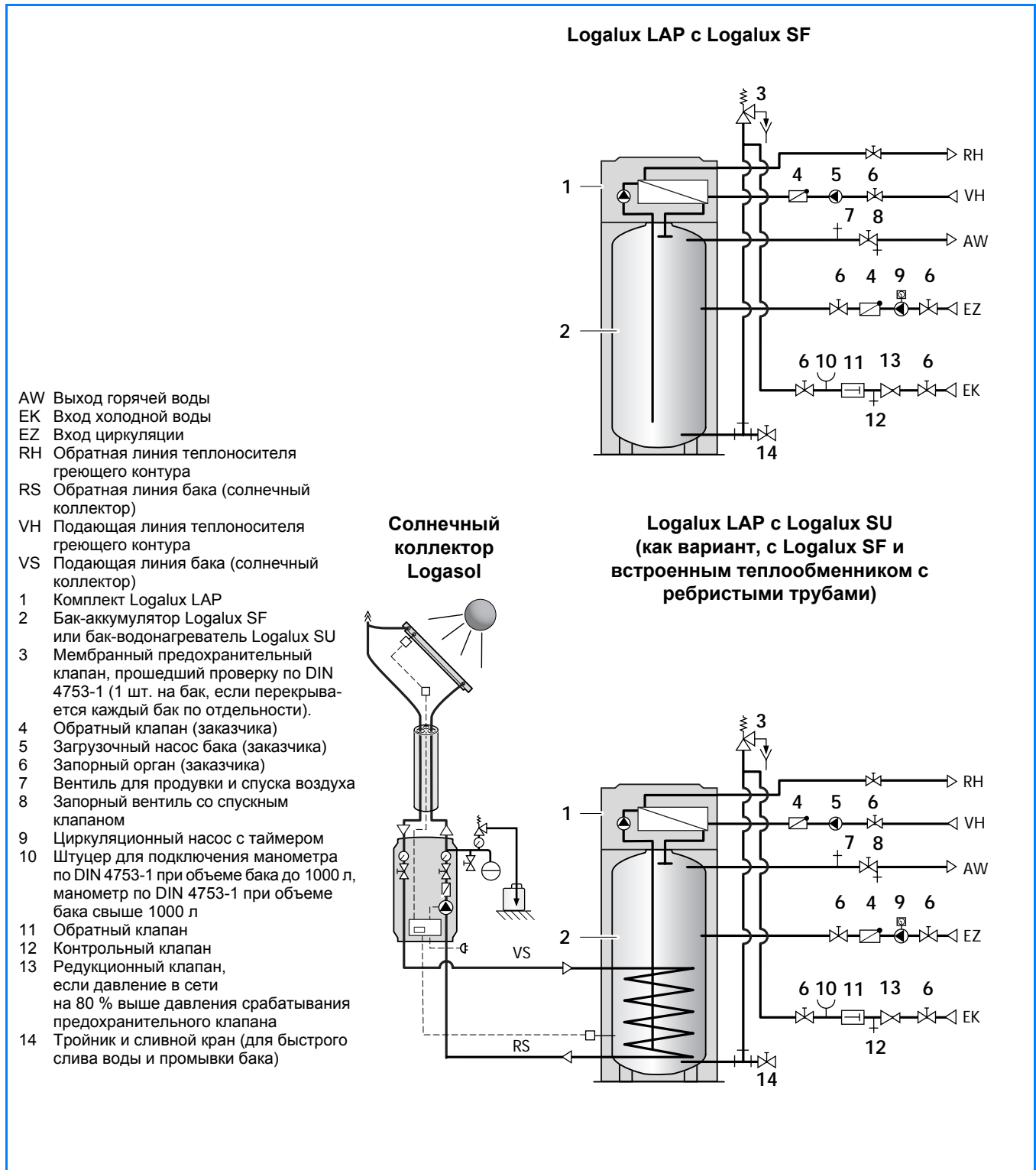
131/1 Гидравлическая схема системы с промежуточным теплообменником: комплект Logalux LAP с баком-водонагревателем Logalux SU или с баком-аккумулятором Logalux SF, подключения бака → стр. 96 и стр. 98
