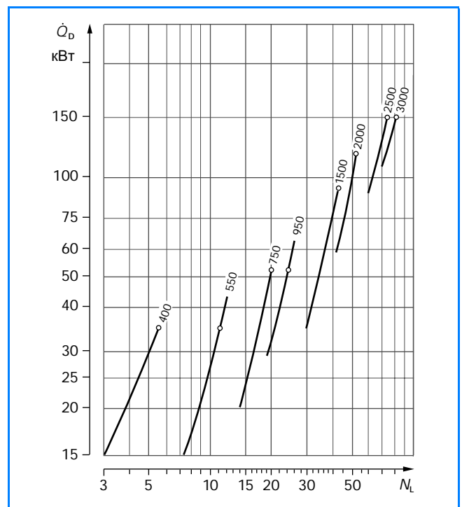
122/3 Зависимость показателя мощности N_L от длительной мощности по горячей воде (о = документация AGFW, → таблица 115/1)
