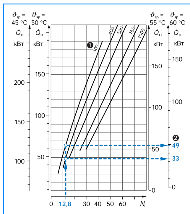
43/1 Аккумуляруемый объем Logalux SF300 - SF1000 в загрузочной системе с промежуточным теплообменником в зависимости от показателя мощности N_L , длительной мощности и температуры воды в баке при использовании загрузочного насоса горячей воды, работающего в прерывистом режиме (...); пример выделен синим цветом (оригинал \rightarrow 129/2)
