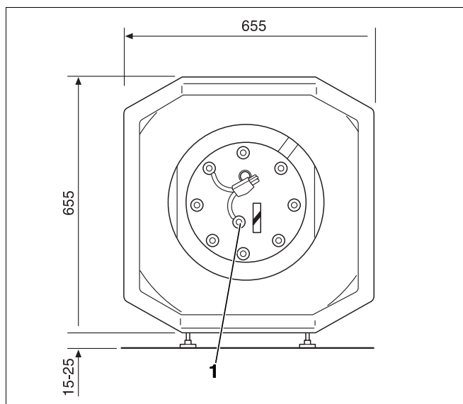
Рис. 2 Размеры
