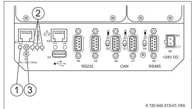
Рис. 18 Переключатели и светодиодная LED сигнализация на панели соединений
