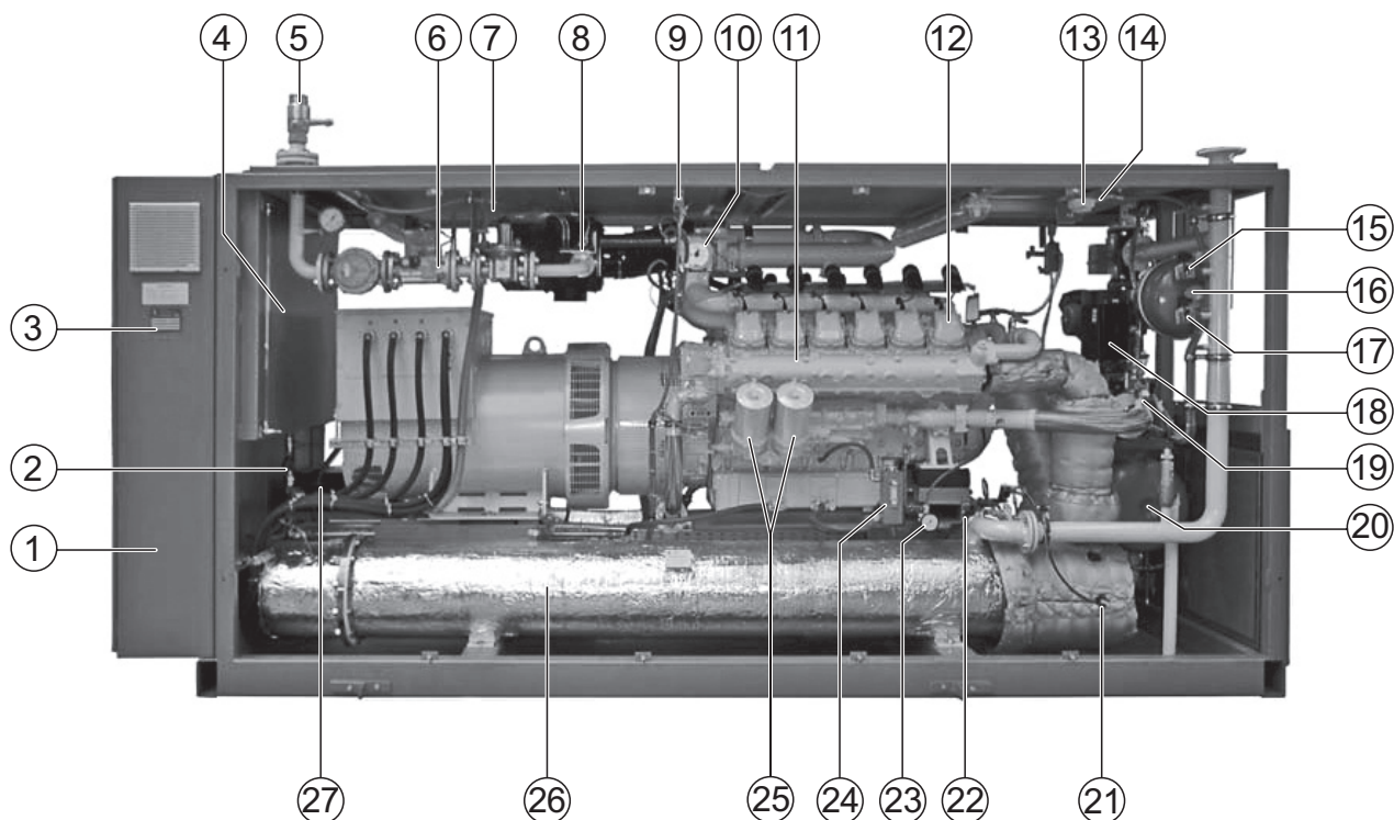
Рис. 1 Loganova EN240 – вид спереди
