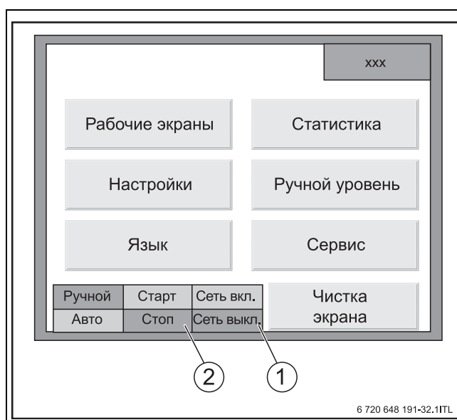
Рис. 13 Выключение установки
