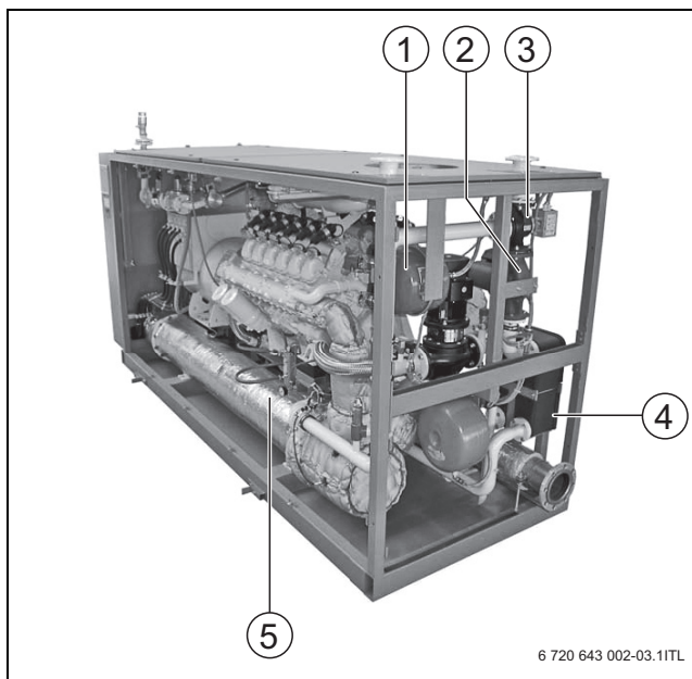
Рис. 3 Отопительный контур и компоненты блок-ТЭС
