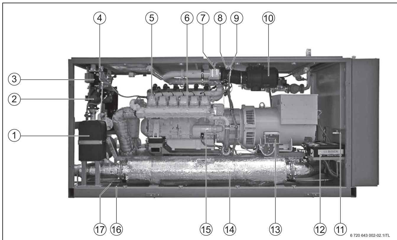
Рис. 2 Loganova EN240 – вид сзади
