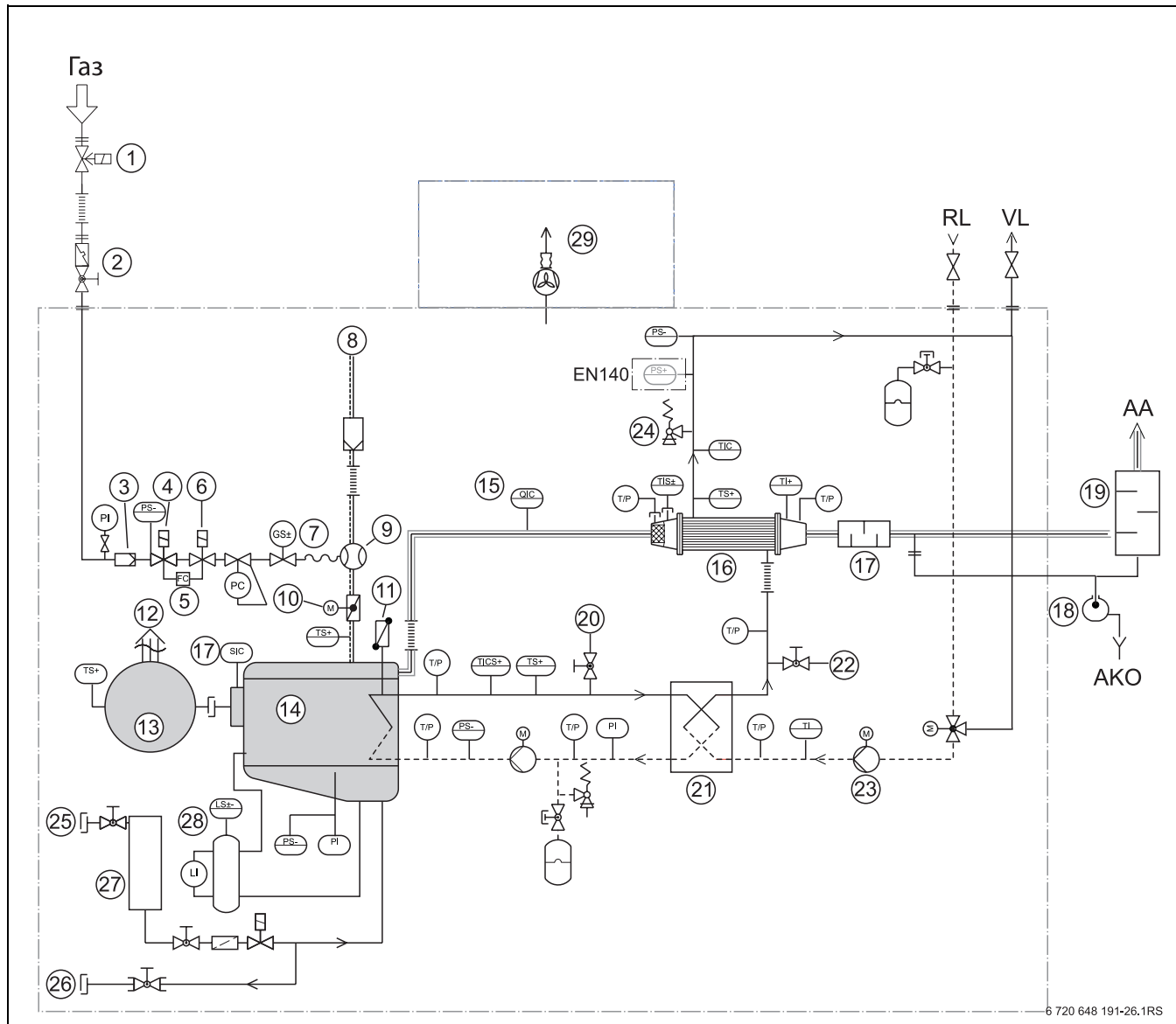
Рис. 6 Функциональная схема EN240 с подключениями
