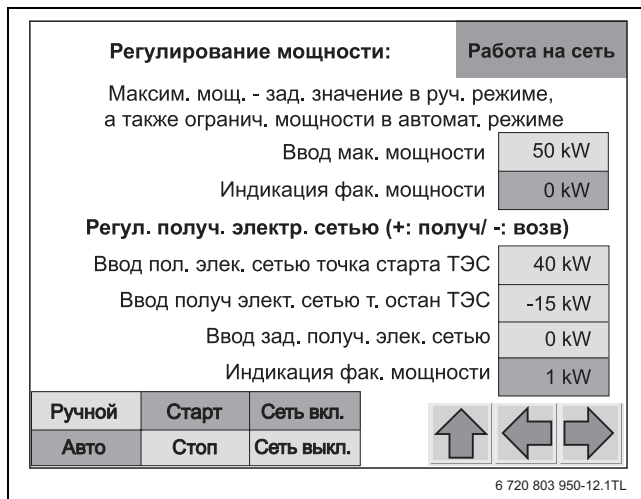
Рис. 26 Экран настройки "Регулирование мощности" (например, с регулированием потребления электроэнергии из сети)
