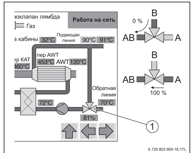
Рис. 32 Направления потоков через трёхходовой клапан
