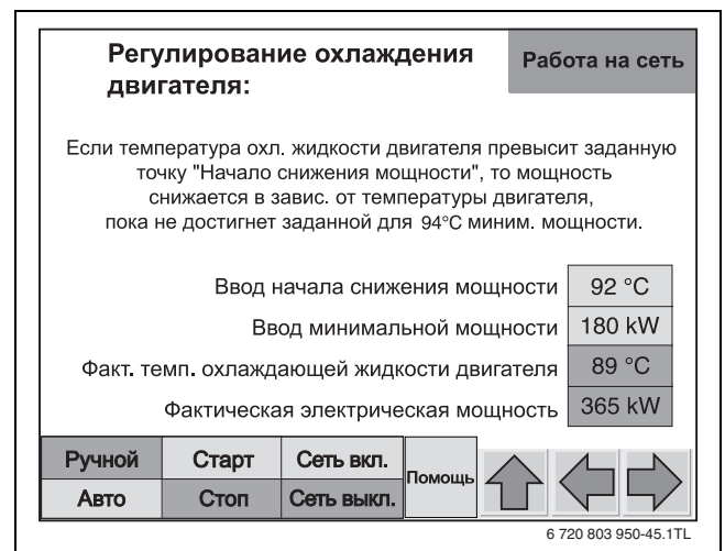
Рис. 27 Экран настройки "Регулирование системы охлаждения двигателя"
