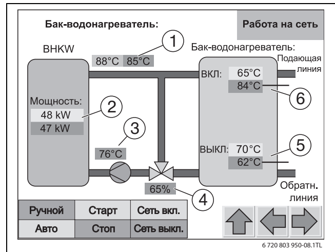
Рис. 12 Рабочий экран "Бак" с 3-ходовым клапаном
