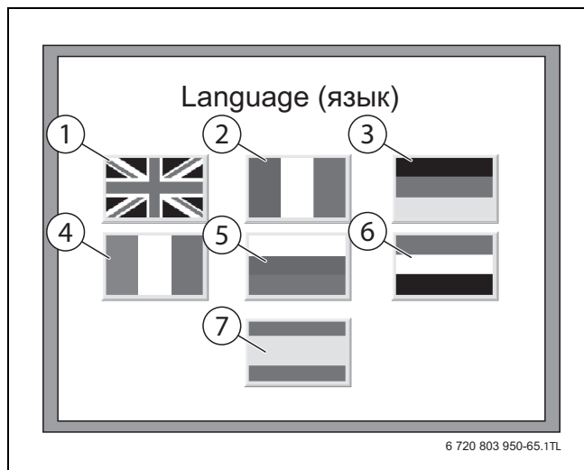
Рис. 53 Подменю "Язык"
