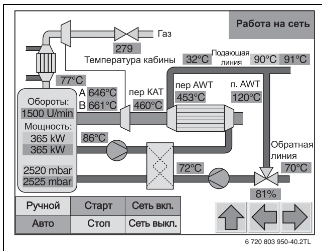
Рис. 11 Рабочий экран "Обзор блок-ТЭС"
