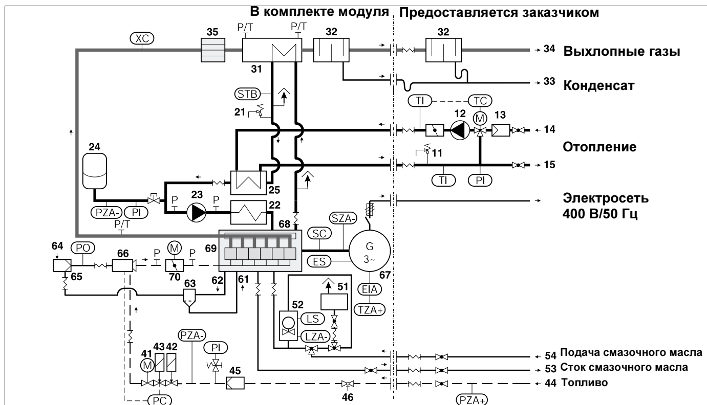
Рис. 2 Устройства контроля
