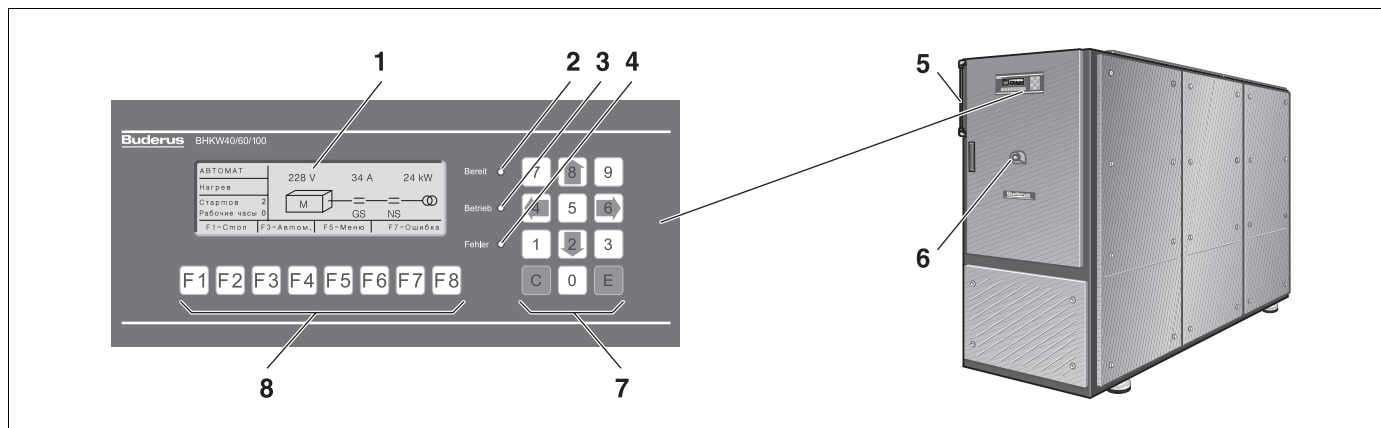
Рис. 1 Панель управления и индикации модуля блок-ТЭС Loganova
