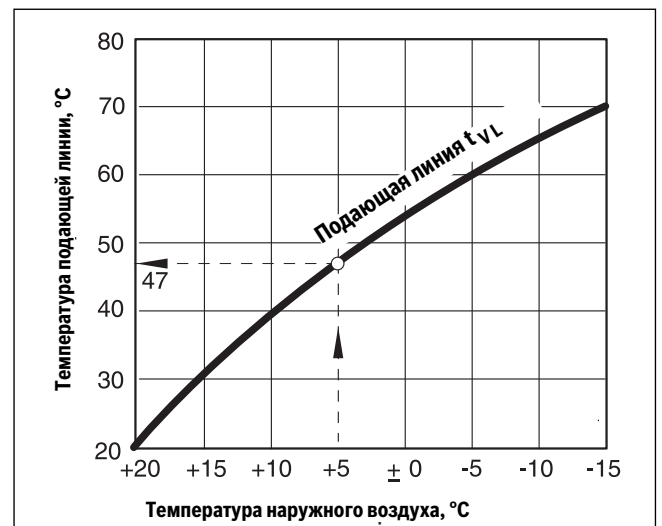
Рис. 3 Графическая характеристика отопительного контура (пример)
