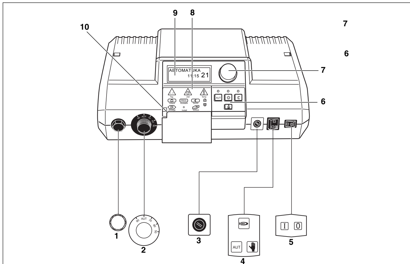
Рис. 4 Элементы управления Logamatic 2107 и Logamatic 2107 M
