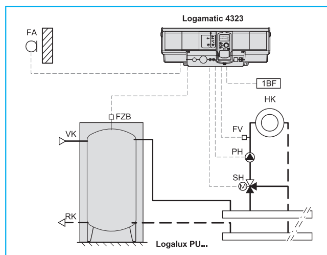
68/2 Пример установки с системой управления Logamatic 4323 в базовой комплектации при использовании её как автономного регулятора отопительного контура (сокращения → Стр. 217)
