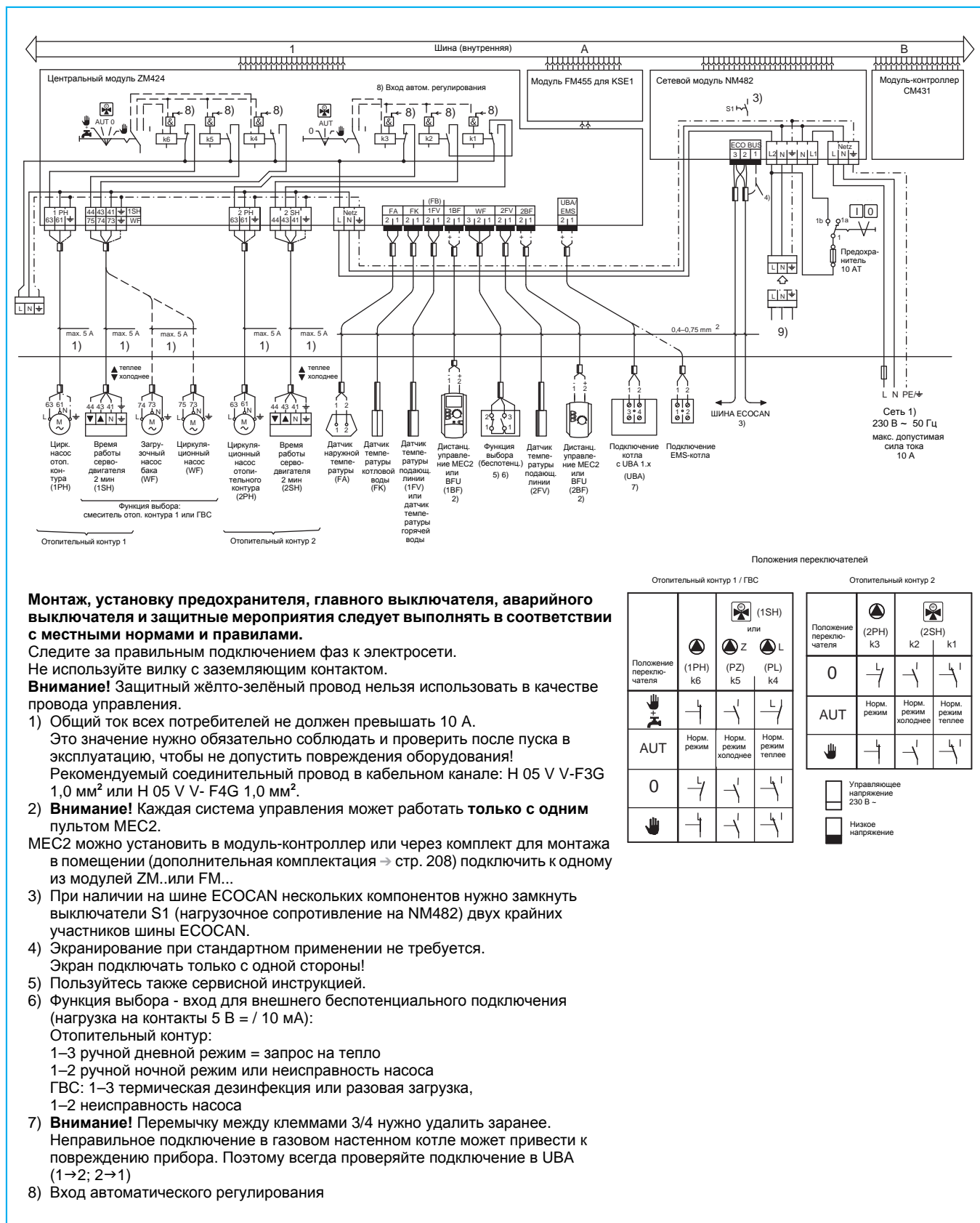
34/1 Электрическая схема системы управления Logamatic 4121 (сокращения → Стр. 217)
