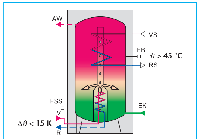
89/3 Нагрев термосифонного бака в соответствии с его температурным расслоением с \Delta\vartheta < 15\text{ K} , но > 5 K при низкой инсоляции (скорость вращения насоса минимум 30 %)
