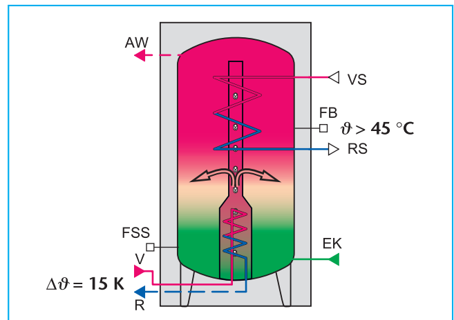
89/2 Нагрев термосифонного бака в соответствии с его температурным расслоением в режиме High-Flow с \Delta\vartheta = 15\text{ K} и высокой переменной скоростью вращения насоса (>45 °C на датчике FB!)
