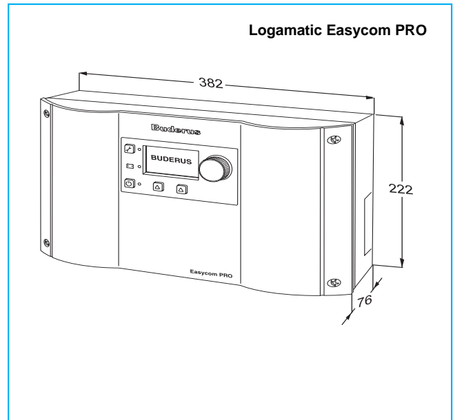
213/3 Размеры модема дистанционной связи Logamatic Easycom PRO
