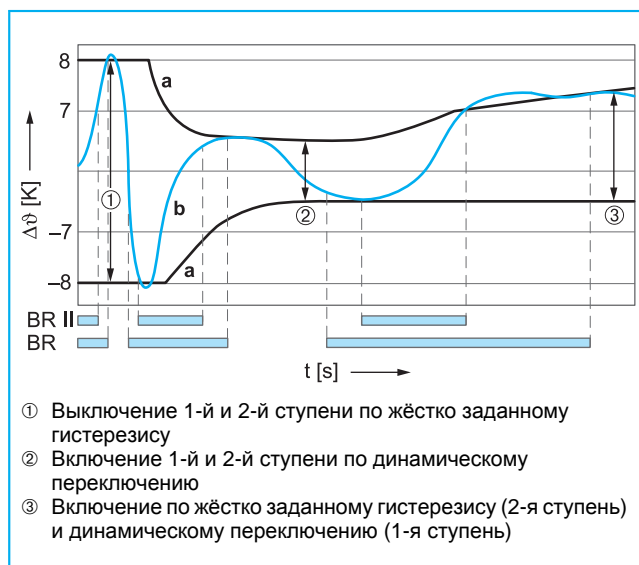
47/3 Диаграмма эффективного (оптимизированного) диапазона переключений
