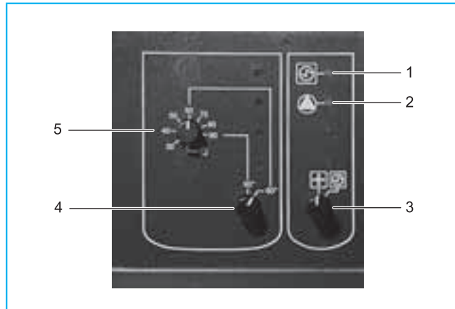
167/2 Центральный модуль ZM429 системы управления Logamatic 4117
