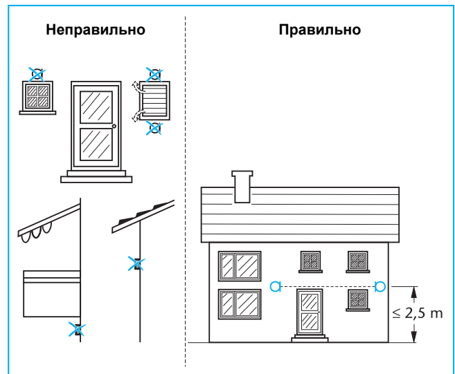
210/1 Расположение датчика наружной температуры
