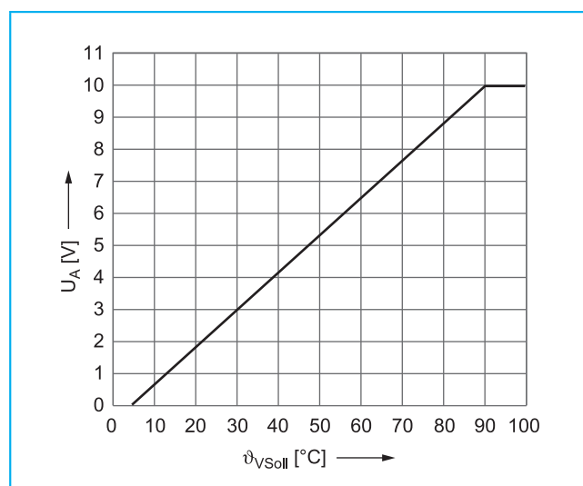
70/2 Выход внешнего заданного значения
