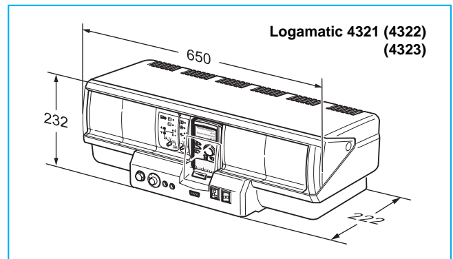
212/4 Размеры цифровых систем управления Logamatic 4321, 4322 и 4323
