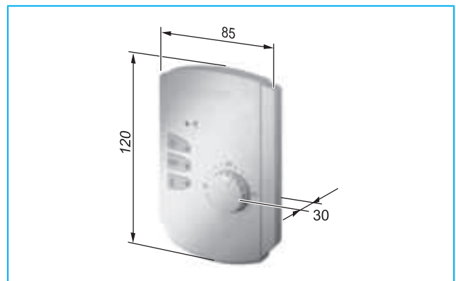
208/2 Дистанционное управление BFU со встроенным датчиком комнатной температуры (BFU/F с приёмником радиосигналов)
