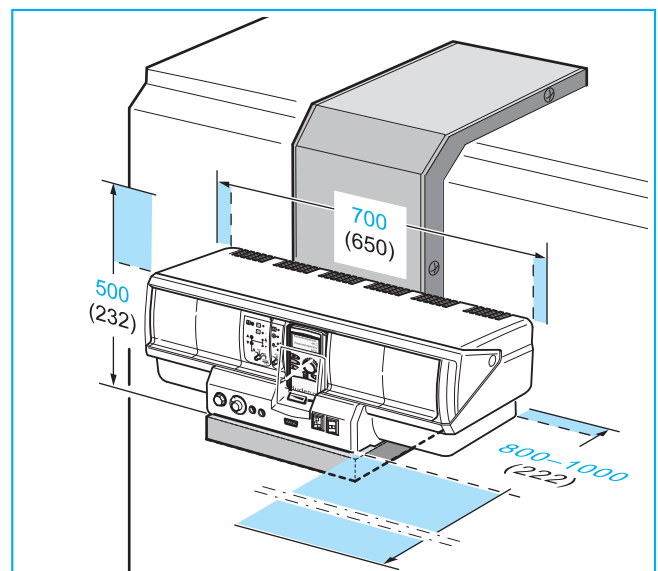
212/6 Минимальная площадь, занимаемая Logamatic 4321 и 4322 при монтаже на кронштейне для бокового крепления 1) системы управления (в скобках приведены размеры системы управления в мм)
