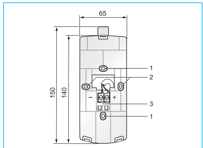
208/3 Настенный держатель для пульта дистанционного управления MEC2
