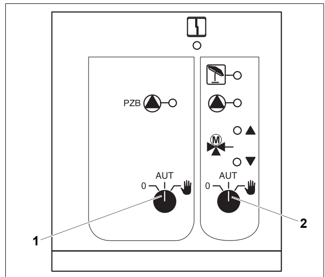
Рис. 26 Центральный модуль ZM433
