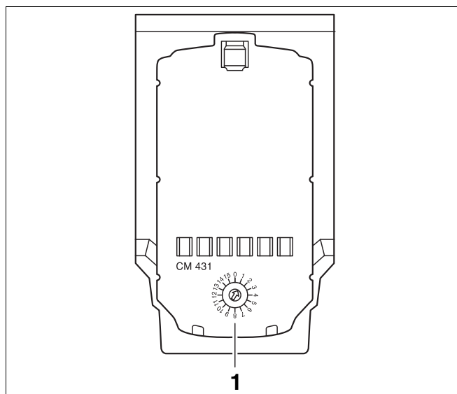
Рис. 5 Настройка адресов
