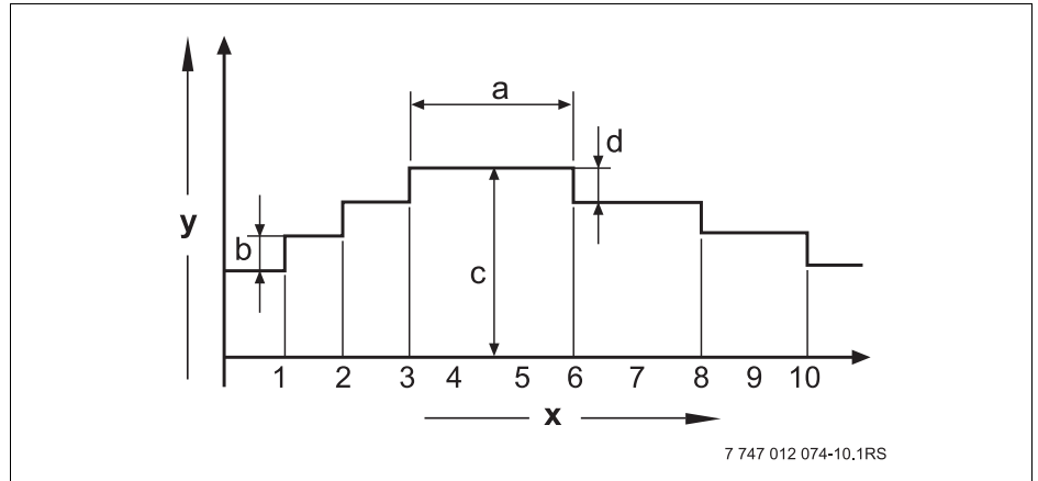
Рис.17 Сушка пола
