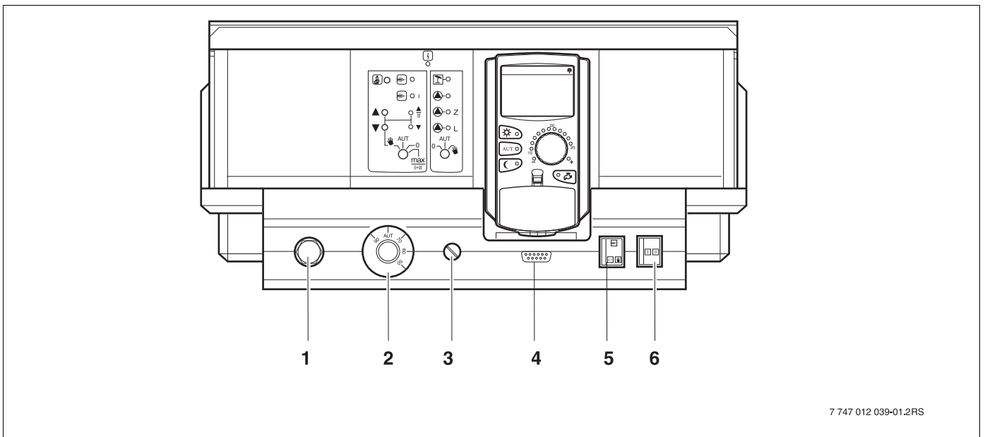
Рис. 4 Система управления Logamatic 4211 (состояние поставки)
