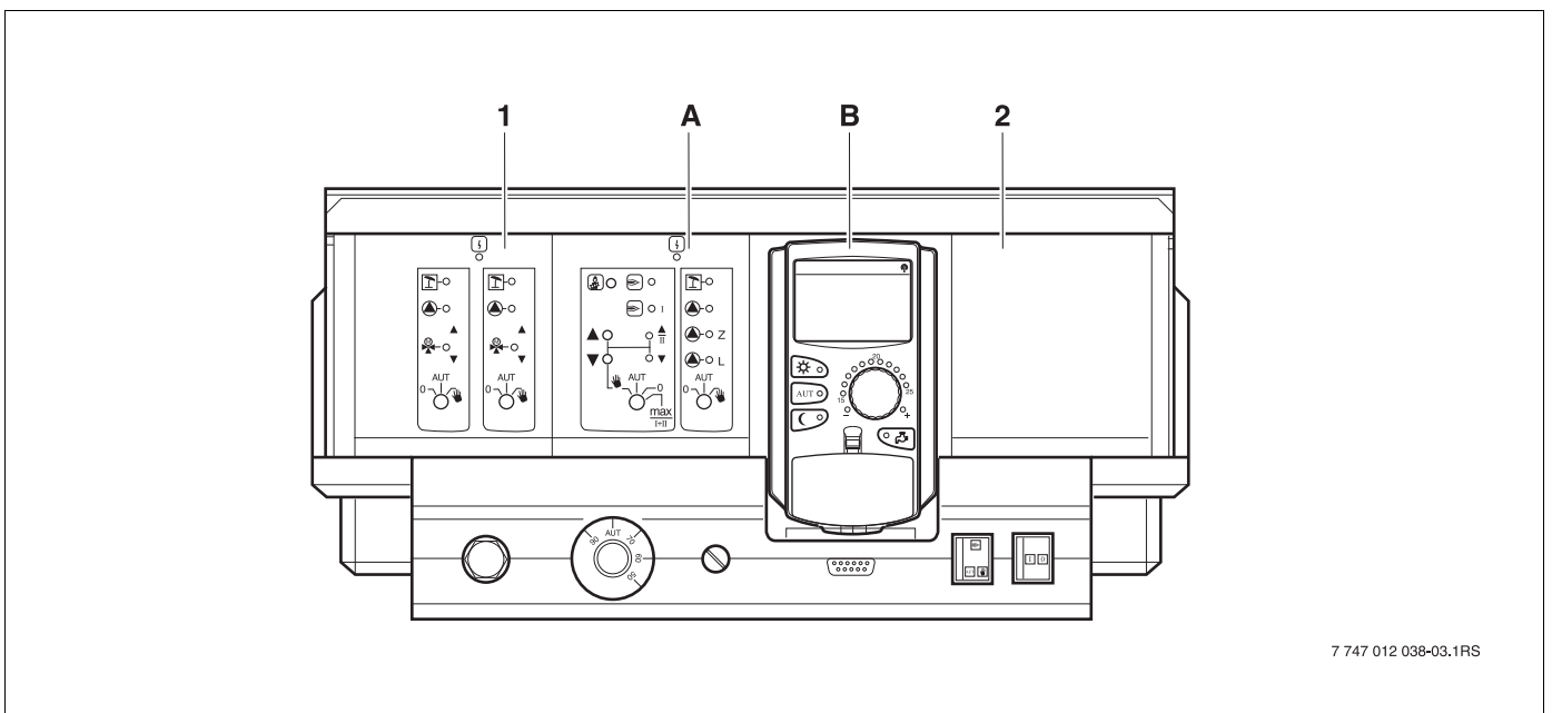
Рис. 5 Комплектация модулями
