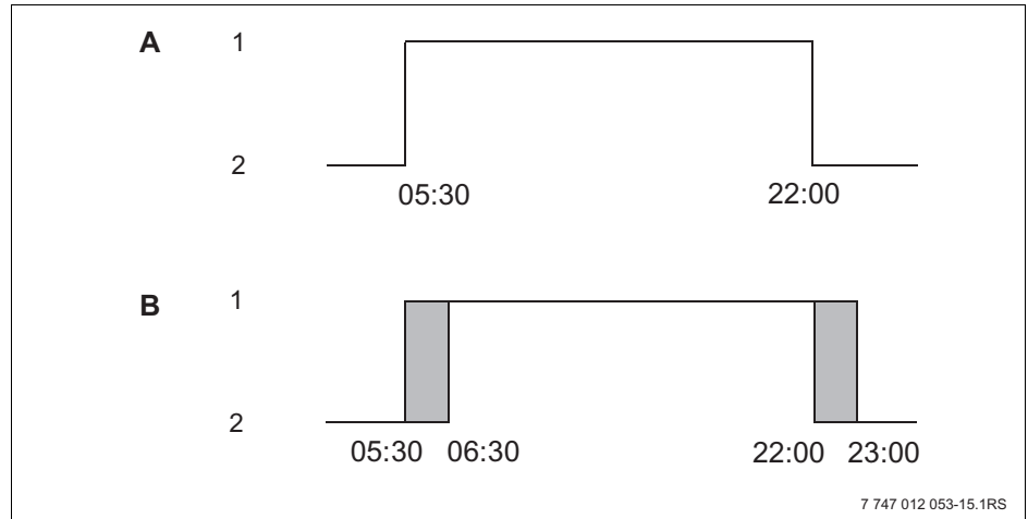
Рис. 14 Изменение времени включения с 05:30 на 06:30 и времени выключения с 22:00 на 23:00 (пример)
