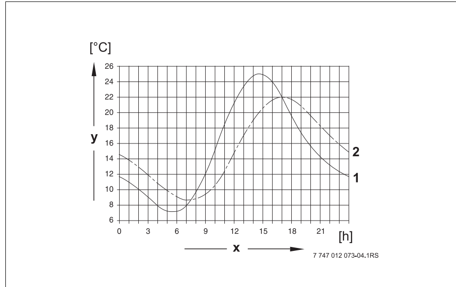
Рис. 15 Сравнение текущей и демпфированной температуры наружного воздуха
