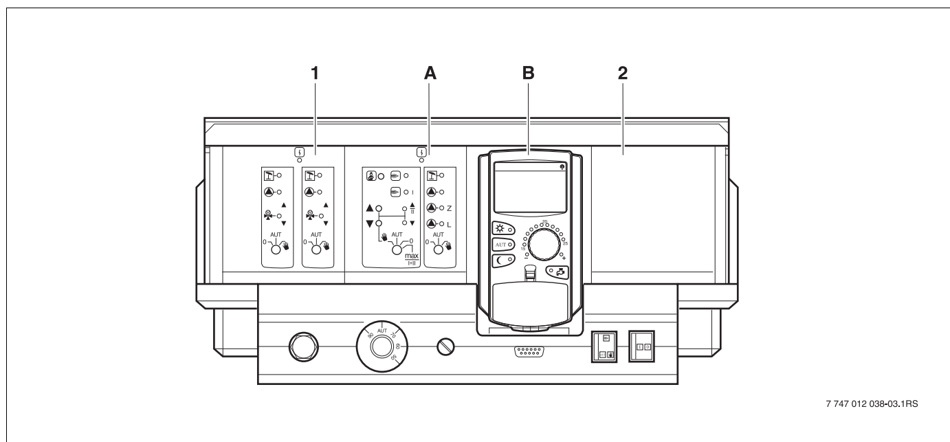
Рис. 5 Комплектация модулями
