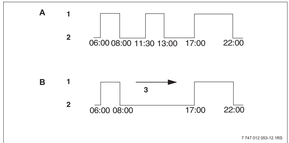
Рис. 18 Отмена отопительного периода
