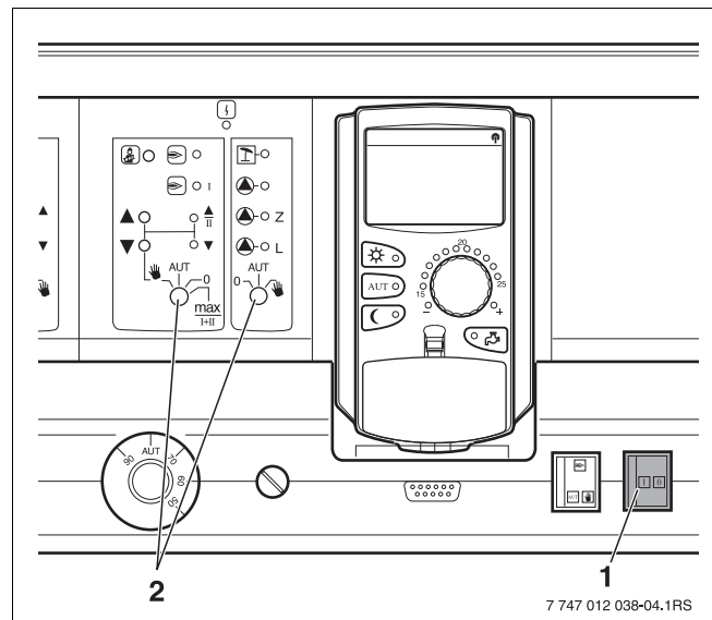
Рис. 8 Пусковой выключатель
