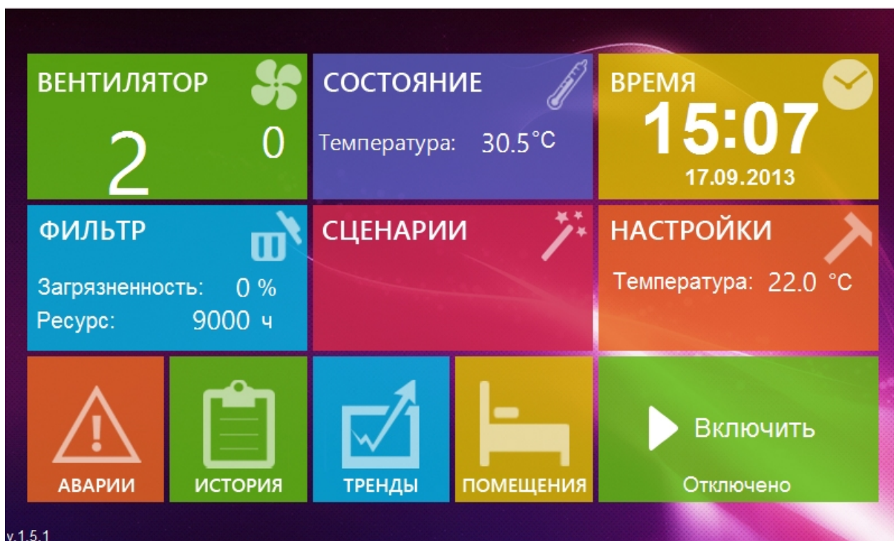
Рисунок 1.1 – Главное окно.
