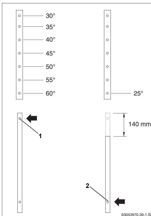
Рис. 12 Выбор угла наклона для вертикальных коллекторов
