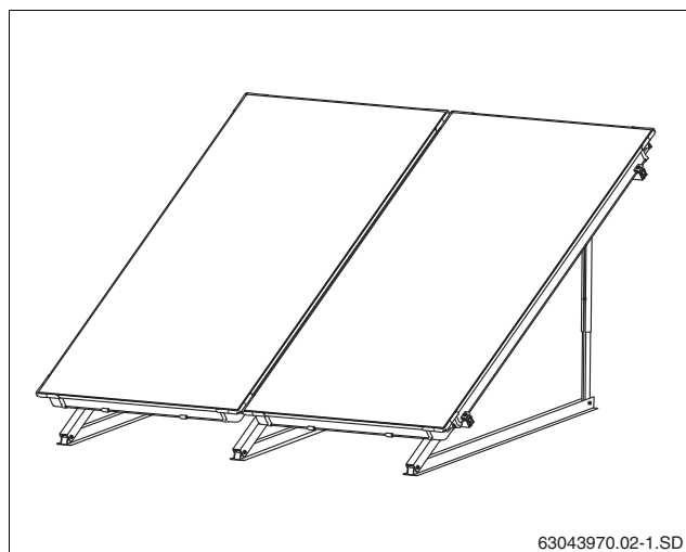
Рис. 37 2 коллектора, установленные на плоской крыше
