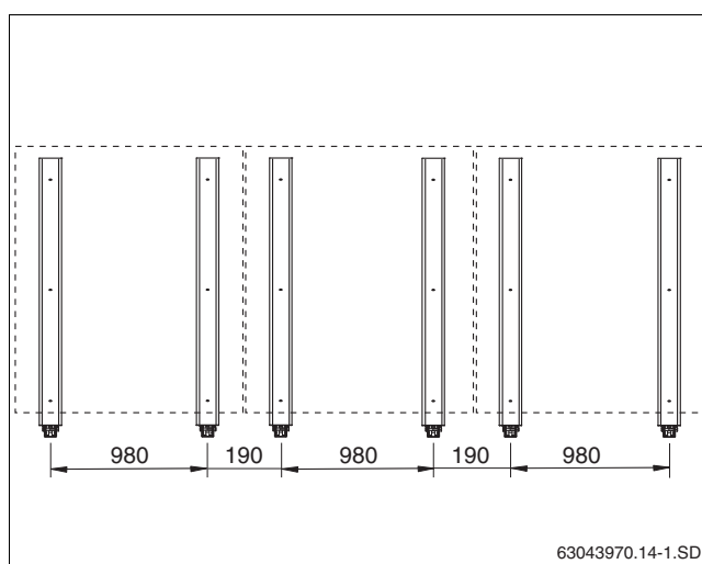
Рис. 25 Исполнение при максимальных нагрузках для 3 вертикальных коллекторов
