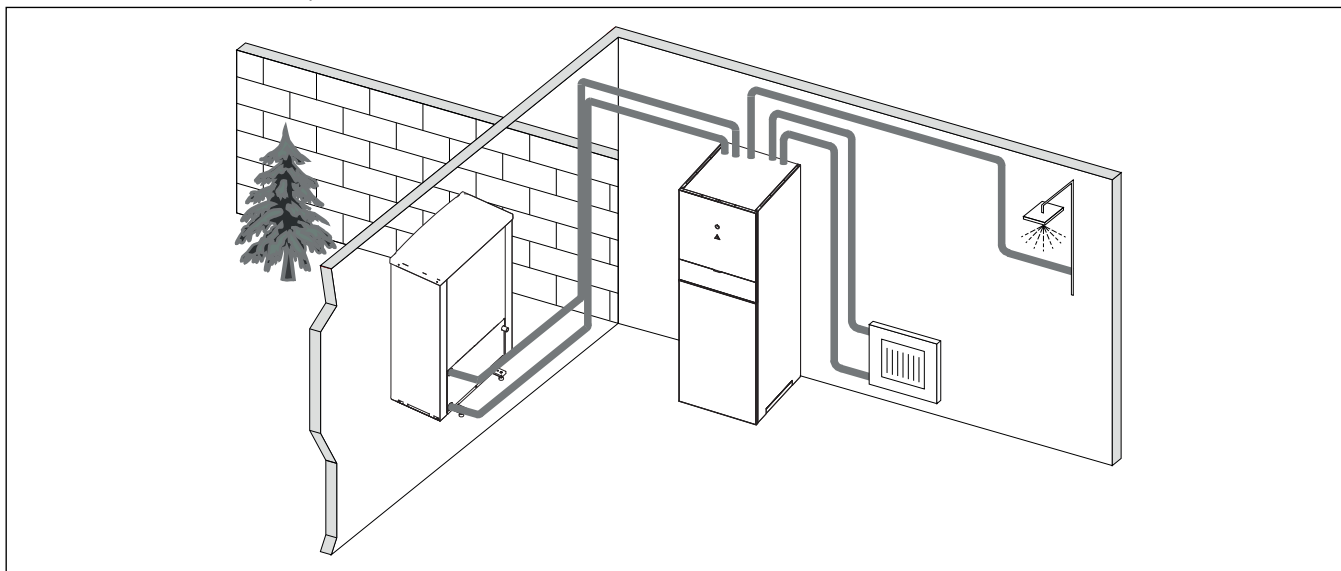
Рис. 3 Тепловой насос Compress 7000i AW, внутренний блок AWM/AWMS со встроенным баком-водонагревателем и дополнительным электронагревателем
