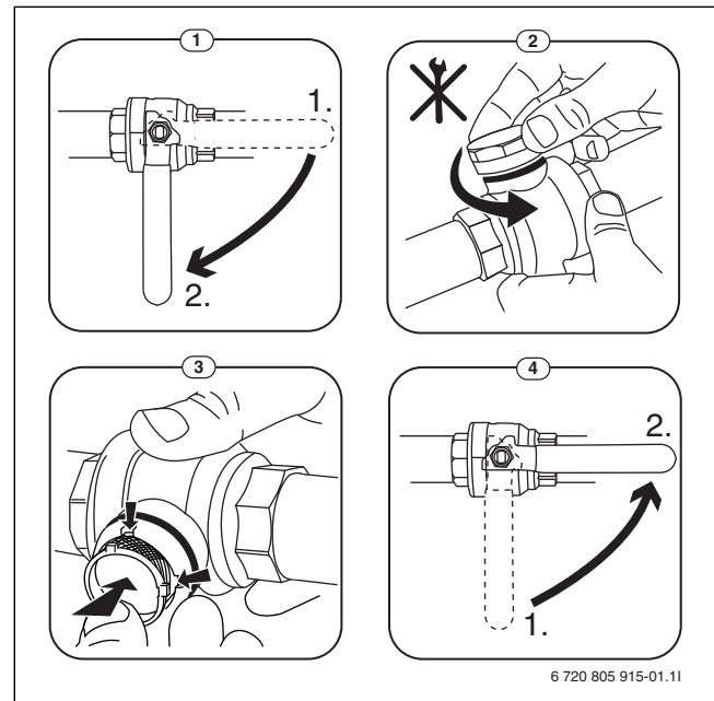
Рис. 7 Чистка сетчатого фильтра
