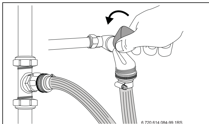
Рис 5 Открыть кран водопроводной воды
