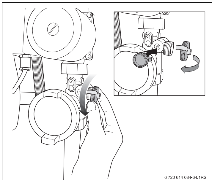
Рис 3 Крышка крана заполнения и слива
