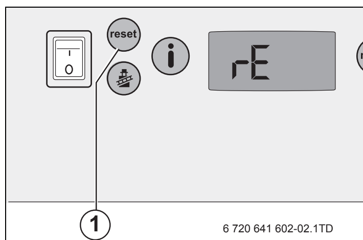
Рис 14 Кнопка „reset“
