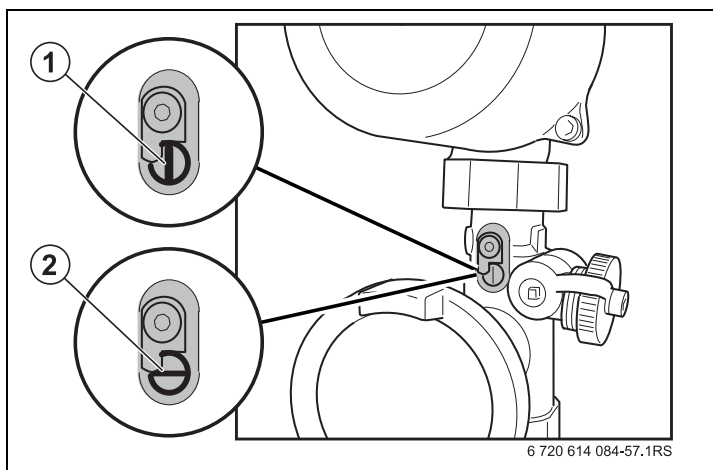
Рис 10 Обратный клапан
