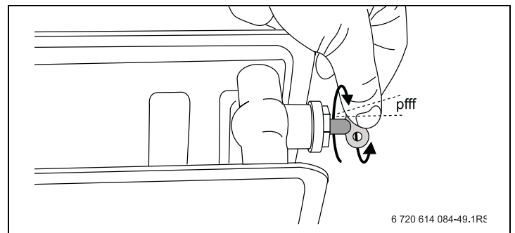
Рис 7 Удаление воздуха из отопительного прибора
