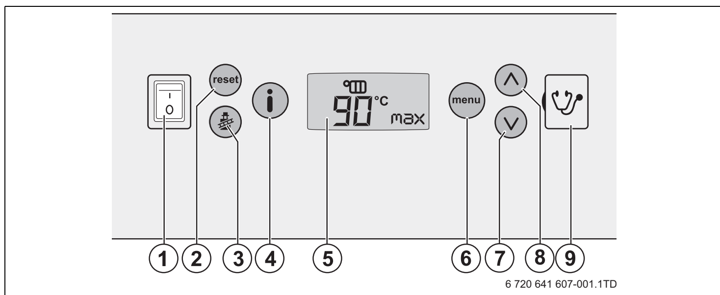
Рис 1 Элементы управления
