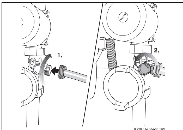
Рис 4 Подсоединение шланга
