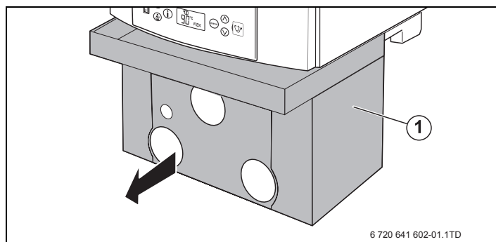
Рис 2 Облицовка группы подключения (дополнительное оснащение)
