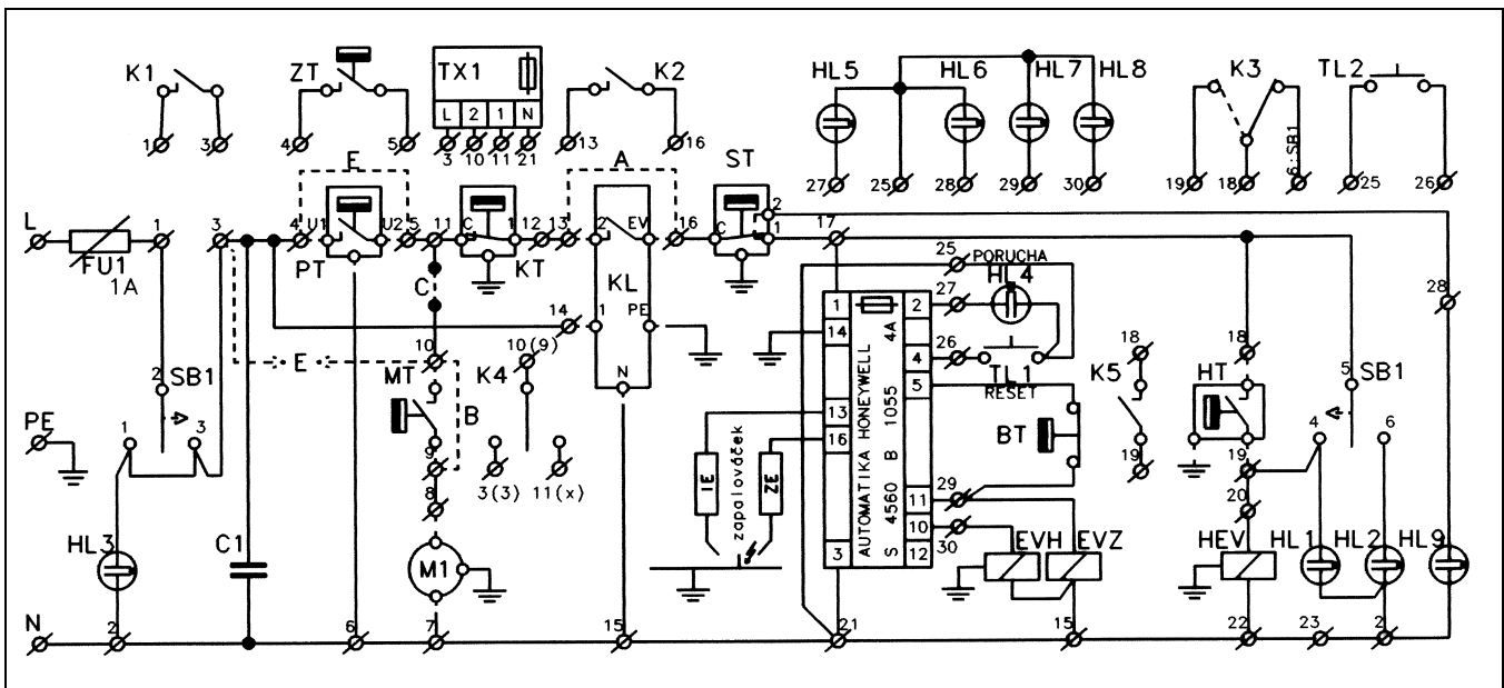
Рис. 12 Электрическая схема котла FN 50 HN
