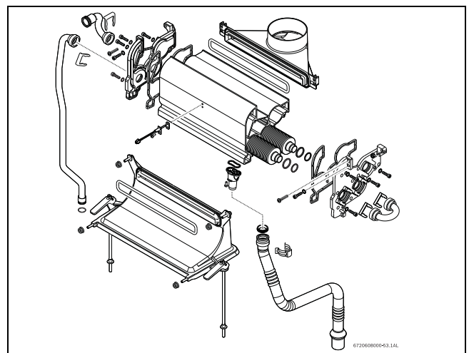
Рис 59 Конденсационный теплообменник
