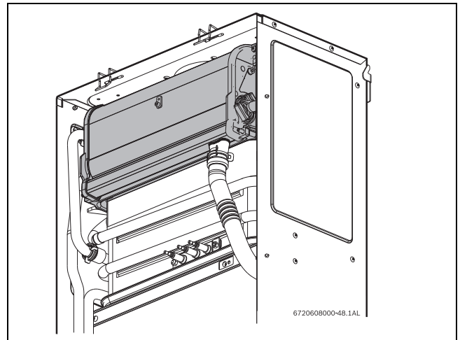
Рис 58 Конденсационный теплообменник
