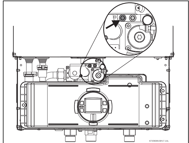
Рис 48 Отверстие для измерения давления газа (левая резьба)
