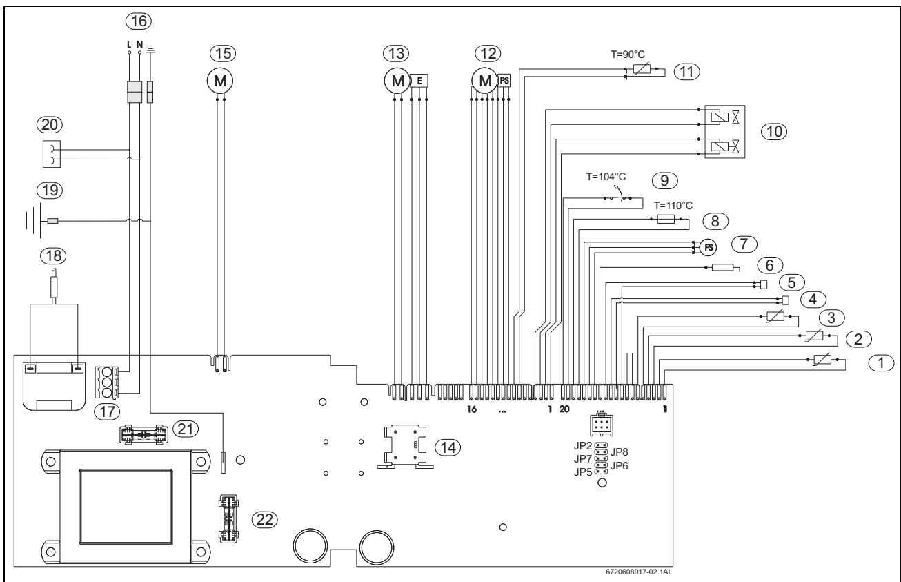
Рис 3 Электрическая схема
