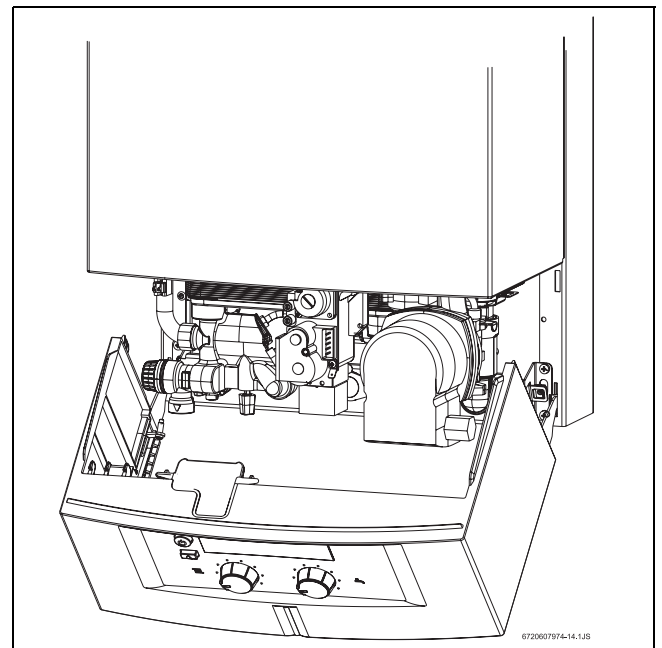
Рис 29 Сервисная позиция для регулирования газа
