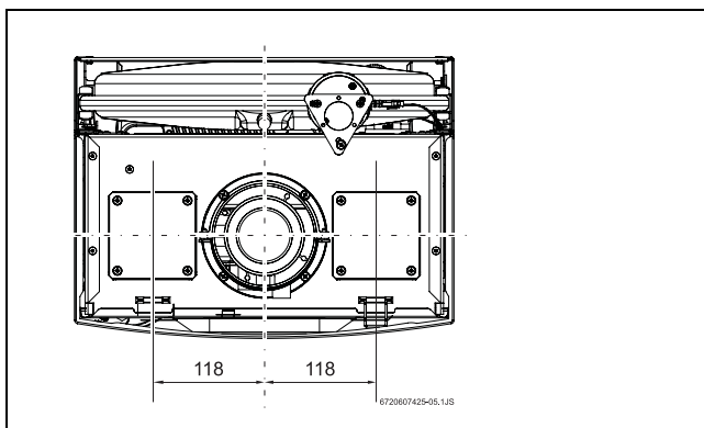
Рис 2 Вид сверху
