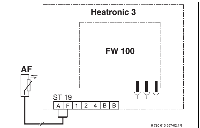
Рис 14 Регулятор встроен с помощью контактов BUS-шины в модуль с Heatronic 3 с подключением к BUS-шине.
