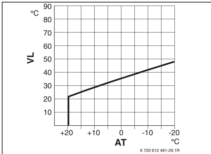
Рис 20 Основная настройка отопительной кривой для подогрева пола
