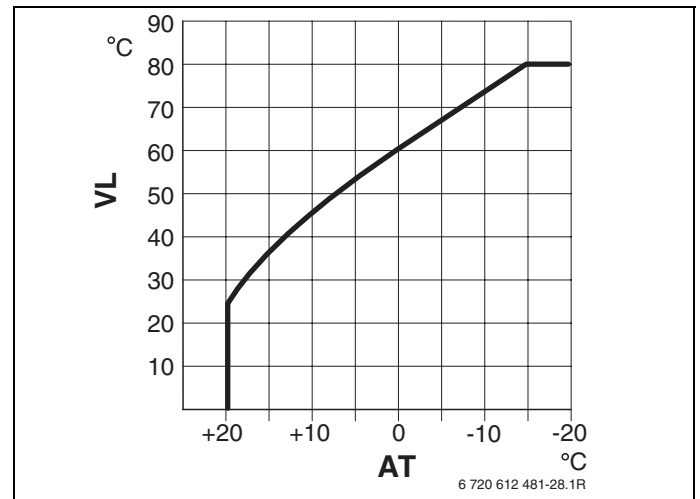
Рис 22 Основная настройка отопительной кривой для подогрева с использованием конвекторов
