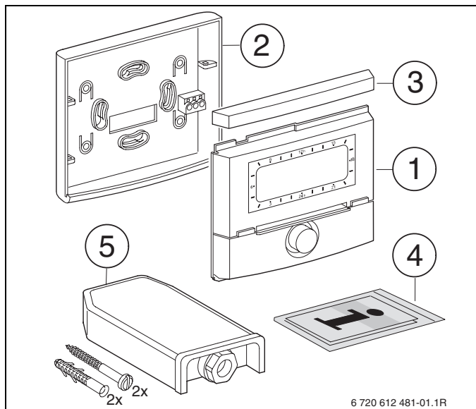
Рис 2 Объем поставки
