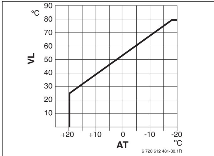
Рис 19 Основная настройка отопительной кривой для метода начальной/конечной точек
