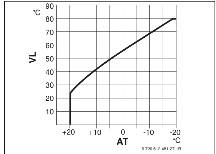
Рис 21 Основная настройка отопительной кривой для подогрева с использованием радиаторов
