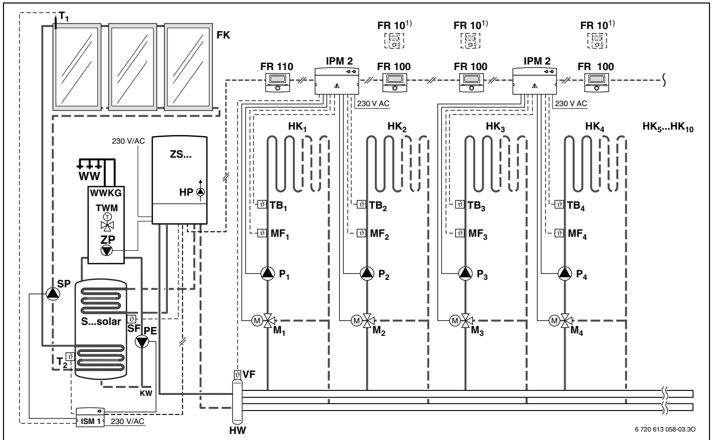
Рис 4 FR 110 и отопительный прибор с подключением бойлера: упрощенная схема (монтажная схема и другие варианты приведены в проектной документации)
