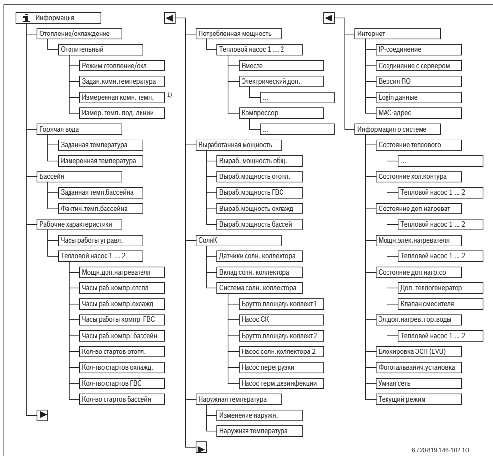
Рис. 5 Структура информационного меню
