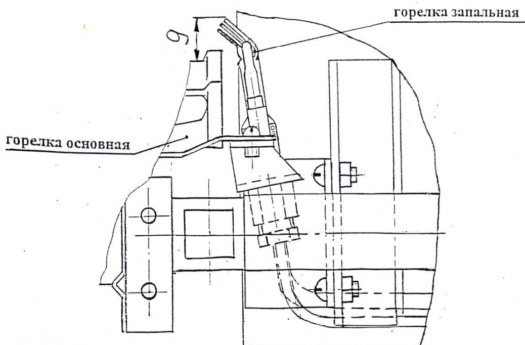
Рис. 7. Схема расположения горелки запальной относительно основной (секционной).
