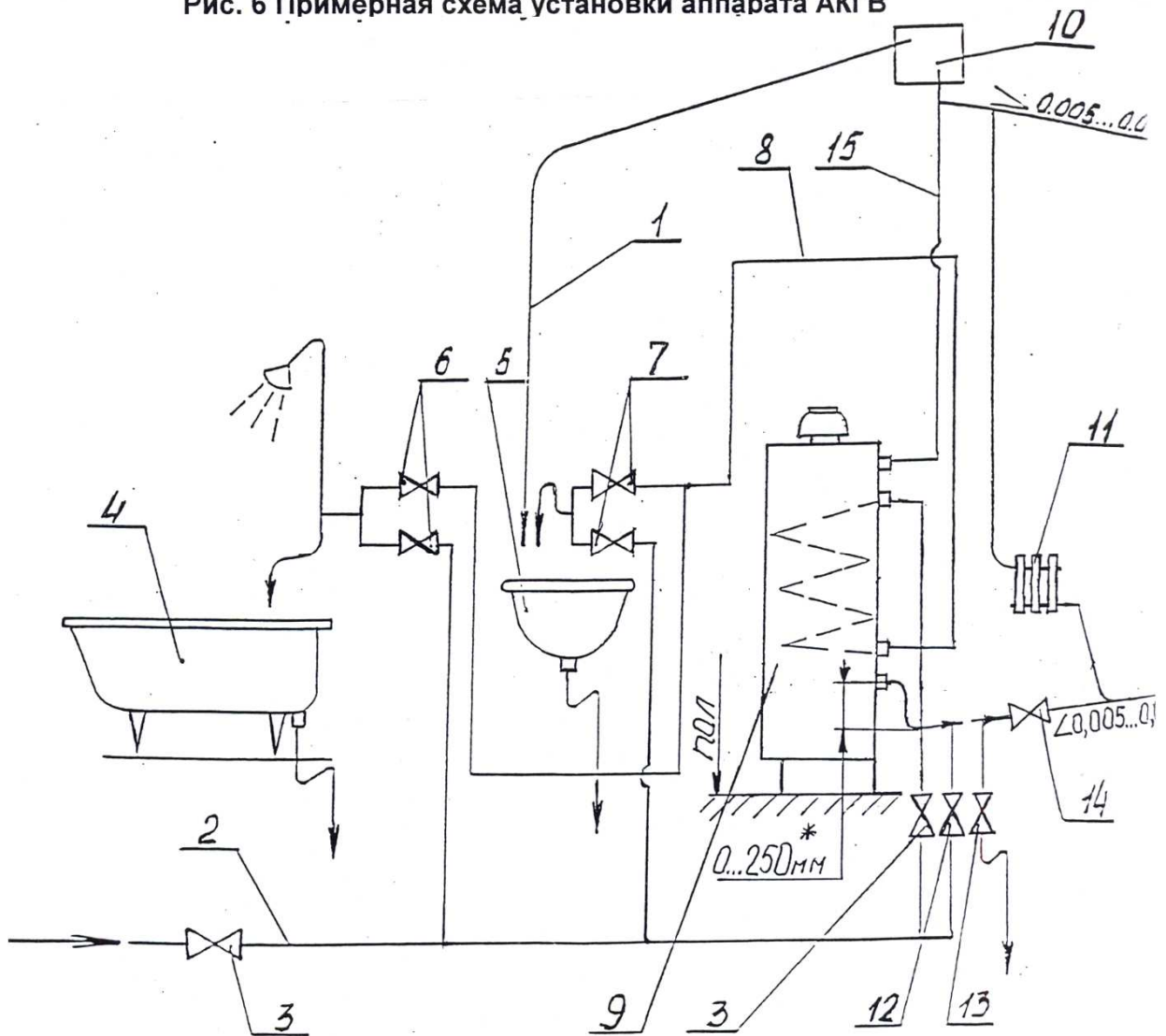
Рис. 6 Примерная схема установки аппарата АКГВ
