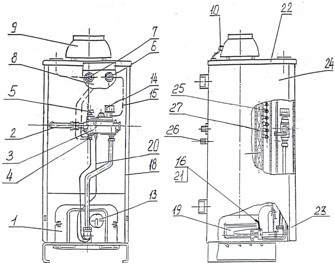
Рис.1. Конструкция аппарата (на виде спереди съёмная панель условно не показана)
