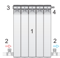
Нижнее подключение
