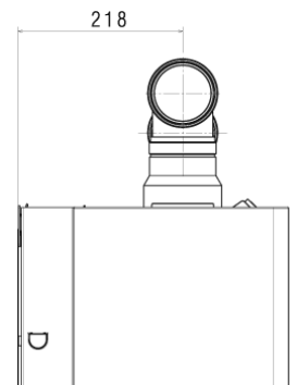
Раздельный воздуховод и дымоотвод
