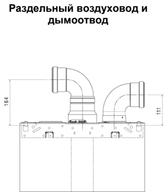
Раздельный воздуховод и дымоотвод
