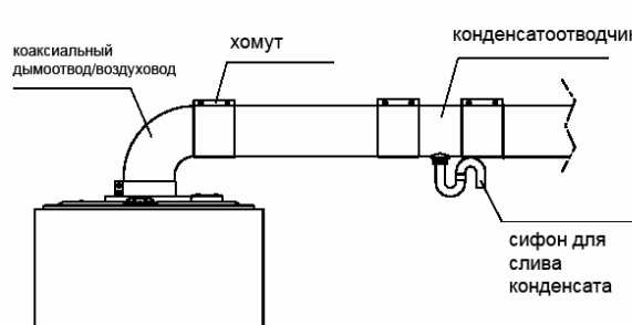
Коаксиальные дымоотвод/воздуховод
