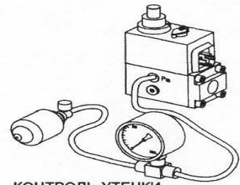
КОНТРОЛЬ УТЕЧКИ
