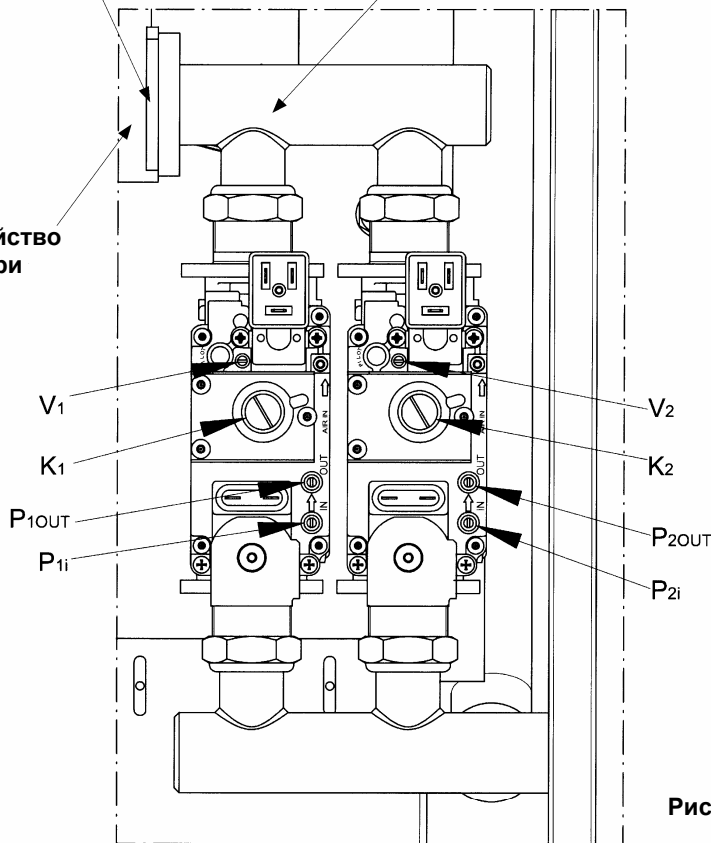
Газовая диафрагма
