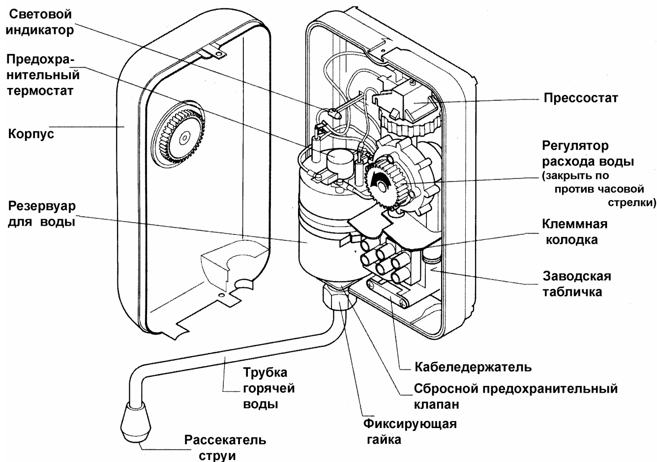
Рис. 1 Устройство водонагревателя
