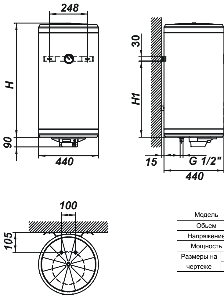
Технические характеристики и размеры, обозначенные на чертеже
