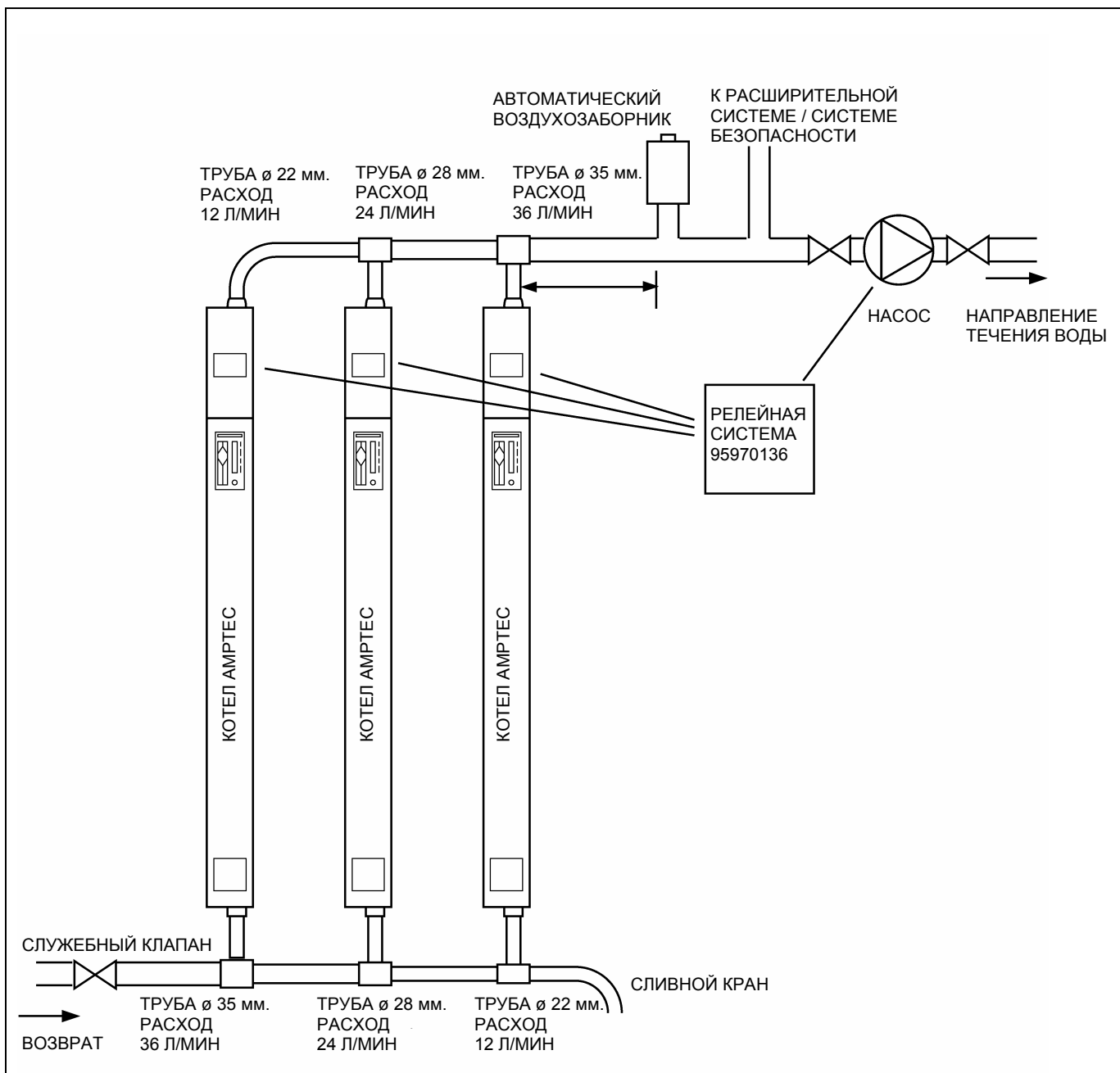
РИС. 4 СХЕМА ВОДОСНАБЖЕНИЯ С ТРЕМЯ КОТЛАМИ
