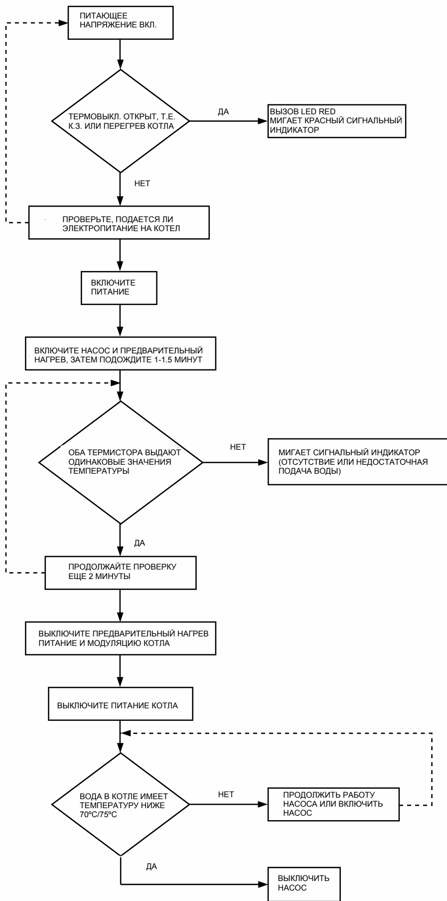
РИС. 12 РАБОТА КОТЛА СЕРИИ С ВЫПУСКА 5
