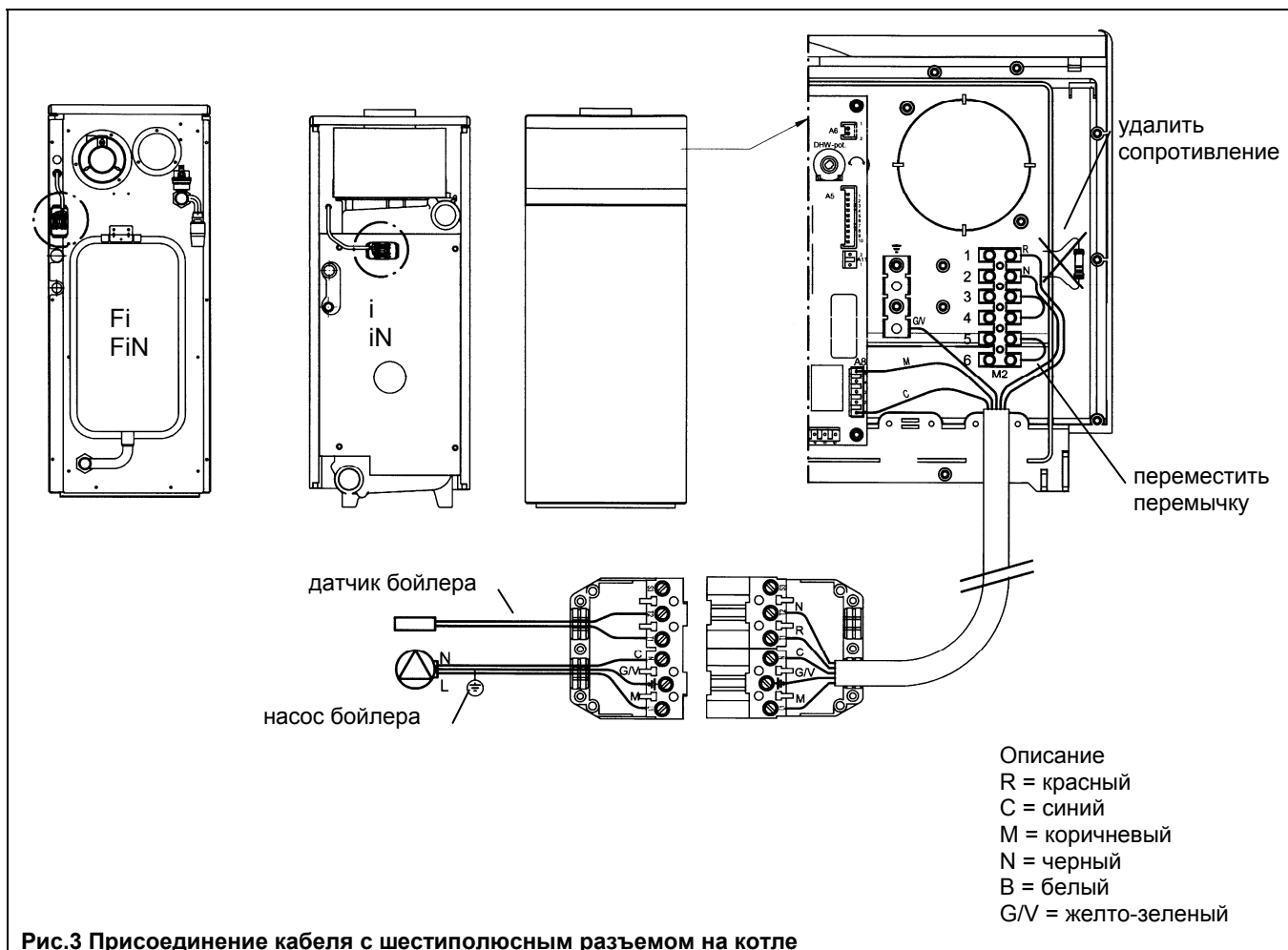
Рис.3 Присоединение кабеля с шестиполосным разъемом на котле
