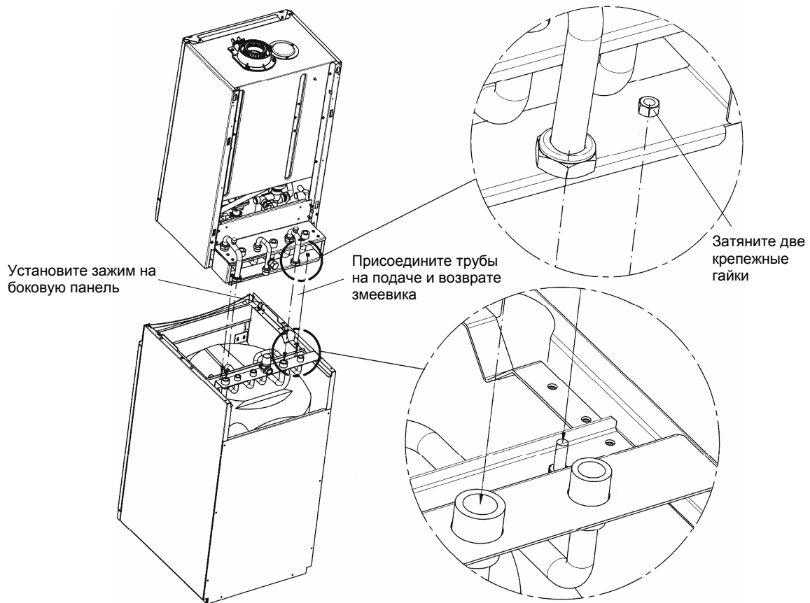
Рис. 1В: Последовательность присоединения бойлера к котлу
