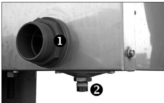
Рисунок 17: Сливная система –вид снаружи
