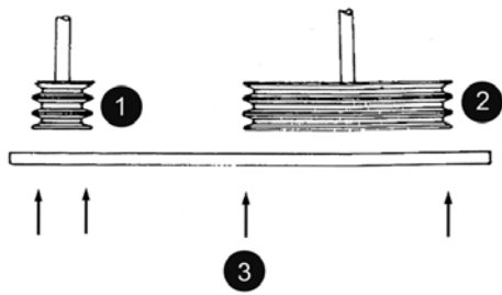
Рисунок 4: Проверка выравнивания шкивов
