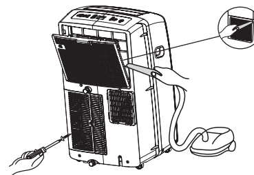
Чистка фильтров с помощью пылесоса
