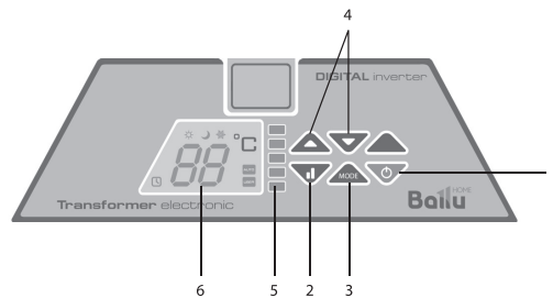
Рис. 2 Панель управления
