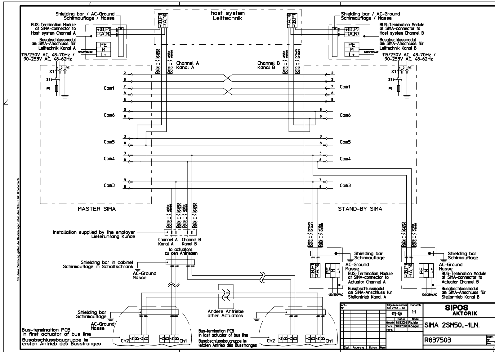
Схема соединений Петлевого дублирования (LOOP REDUNDANCY), т.е. замкнутая петля, 2 Мастер-станции SIMA в режиме HOT-STAND-BY
